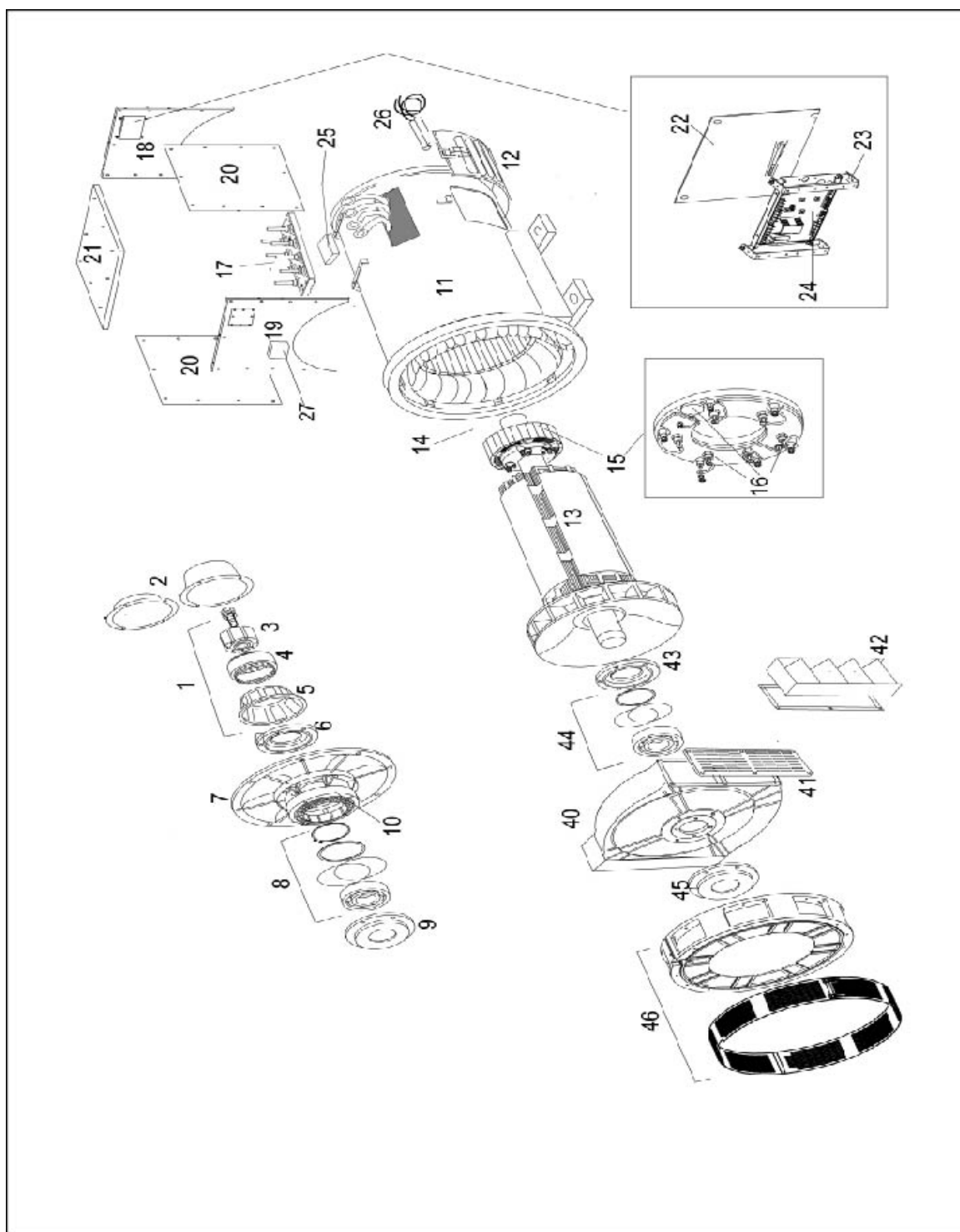
FIGURA 17. ALTERNADOR HC4 DE DOS COJINETES
