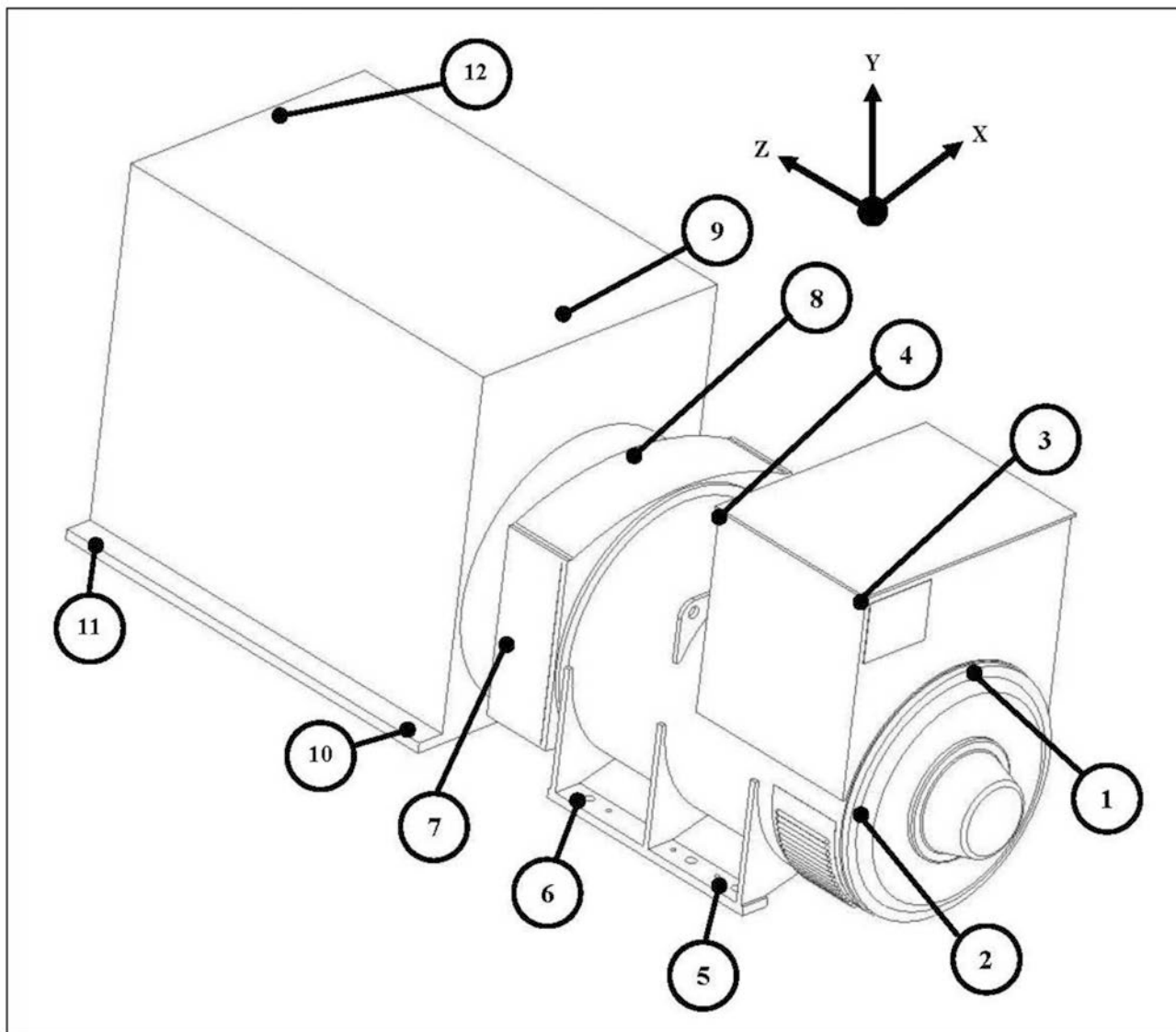
FIGURA 6. UBICACIONES DE MEDICIÓN DE LA VIBRACIÓN
