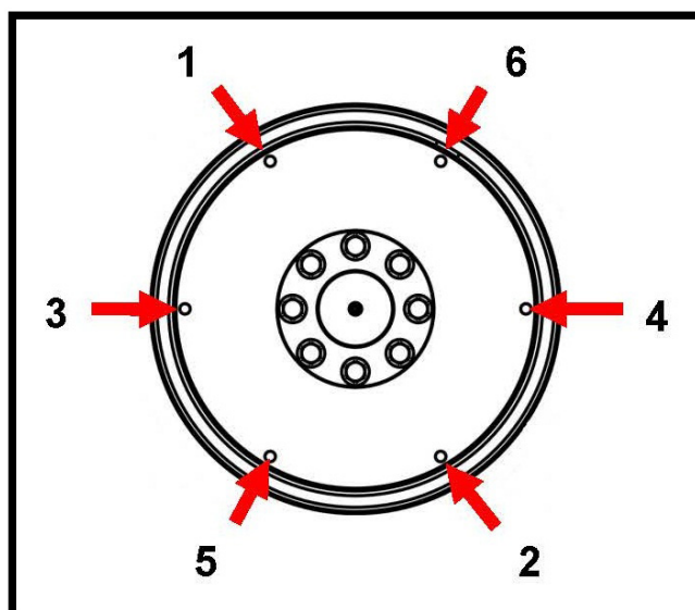
FIGURA 11. SECUENCIA DE FIJACIÓN
