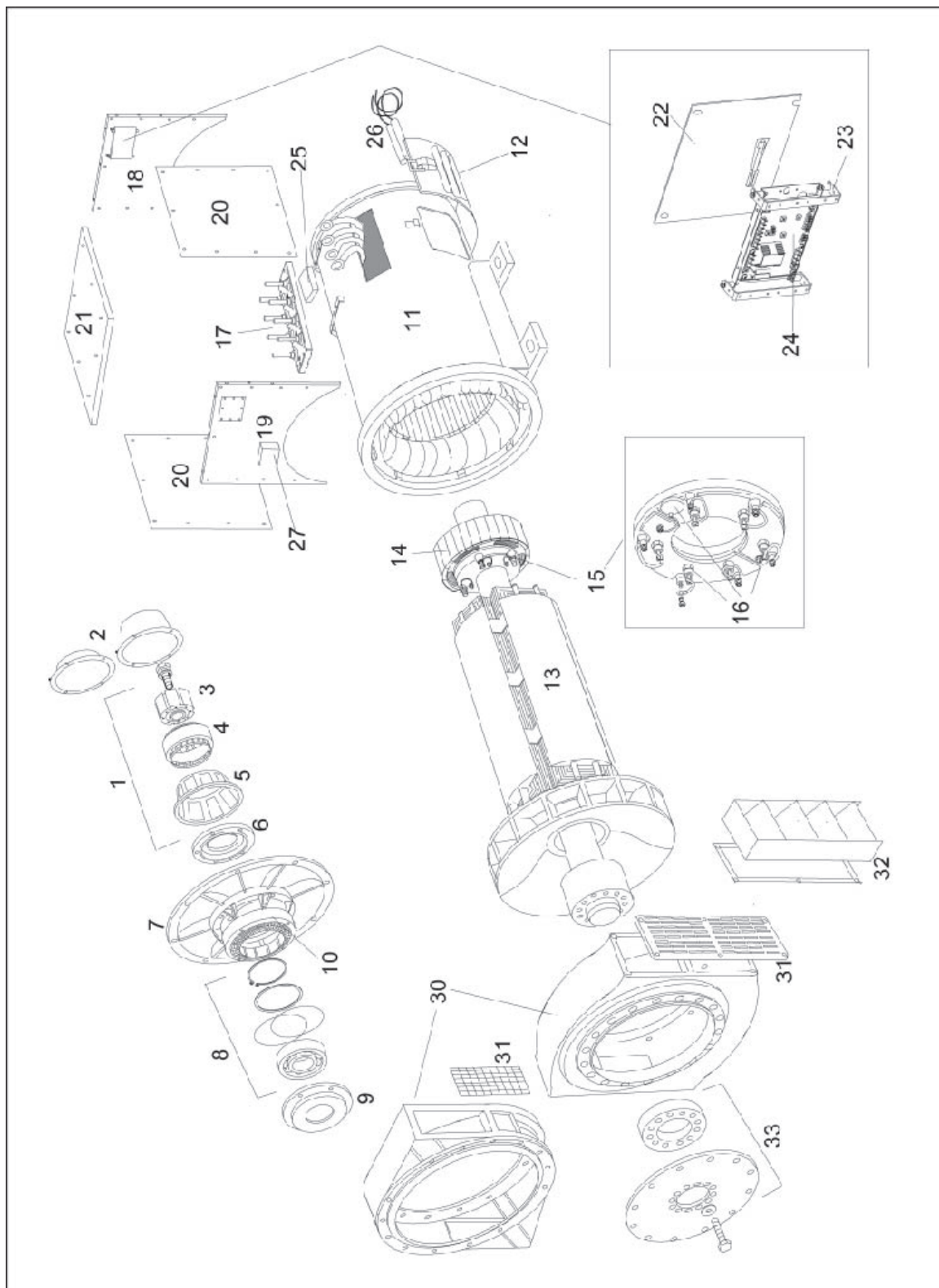
FIGURA 16. ALTERNADOR HC4 DE COJINETE ÚNICO
