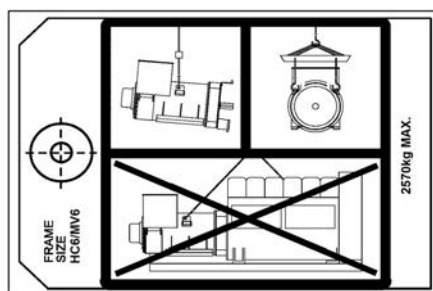
FIGURA 7. ETIQUETA DE ELEVACIÓN
