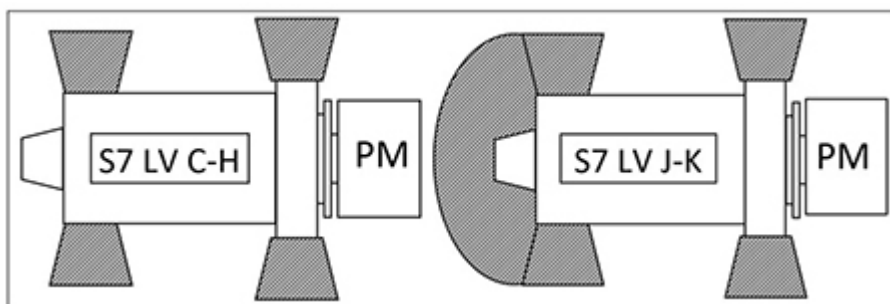
FIGURE 5. ZONES DE DANGER DE L'ALTERNATEUR S7 LV
