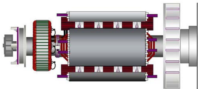
FIGURE 20. ROTOR DE L'ALTERNATEUR À PALIER SIMPLE MONTRANT LES DISQUES D'ACCOUPLEMENT BOULONNÉS À LA COURSE D'ACCOUPLEMENT À L'EXTRÉMITÉ MOTRICE (À DROITE)
