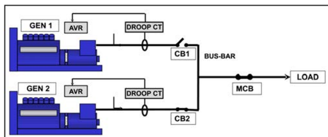
FIGURE 23. ALTERNATEURS PARALLÈLES OU DE SYNCHRONISATION
