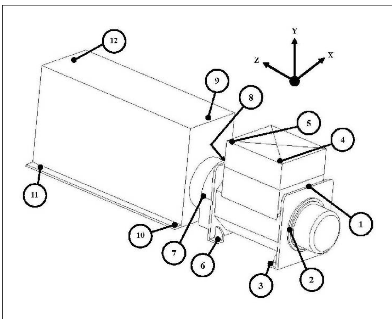
FIGUR 14. VIBRATIONSMÄTNINGSPOSITIONER
