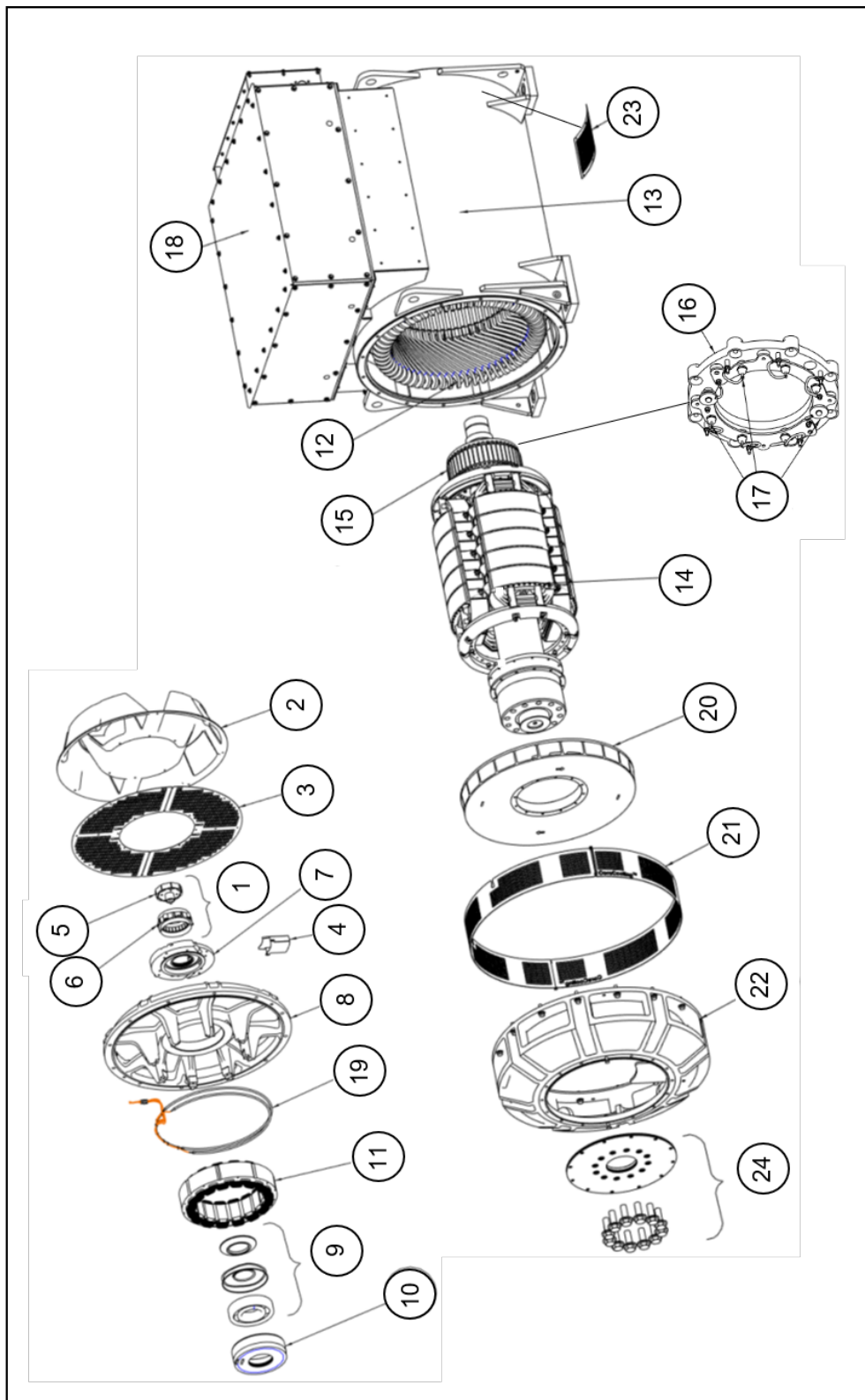
FIGUR 26. S9 VÄXELSTRÖMSGENERATOR MED ETT LAGER
