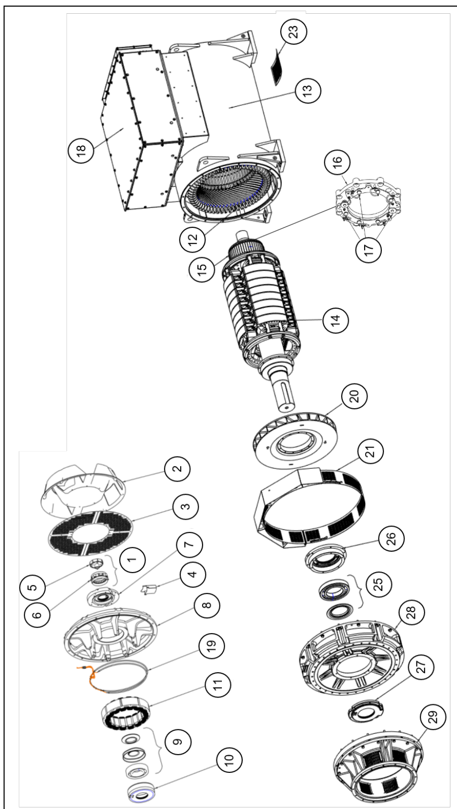
FIGUR 27. S9-VÄXELSTRÖMSGENERATOR MED TVÅ LAGER
