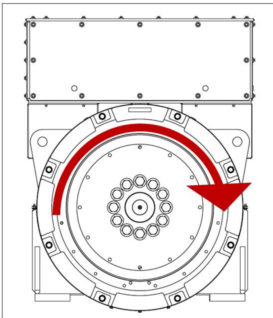
FIGUR 20. ROTATIONSRIKTNING
