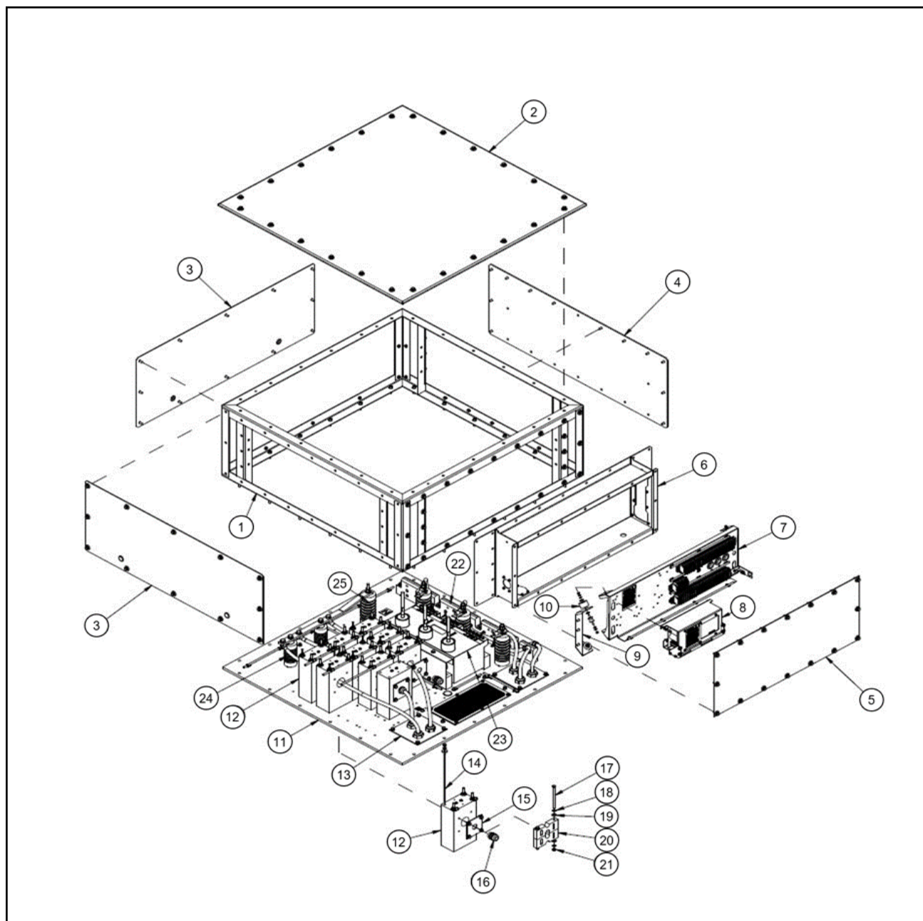
FIGUR 28. TERMINALBOXDELAR OCH -FÄSTEN FÖR MEDELHÖG- OCH HÖGSPÄNNING
