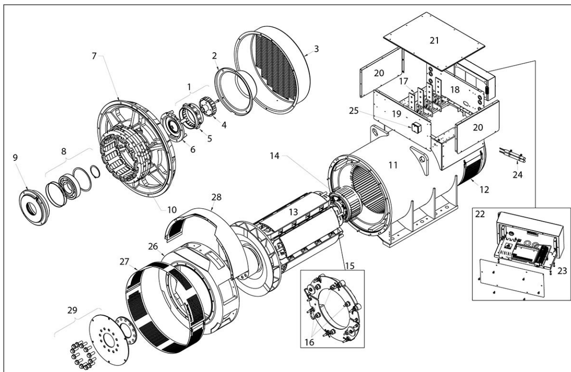
FIGURA 26. ALTERNADOR DE UN SOLO COJINETE A7
