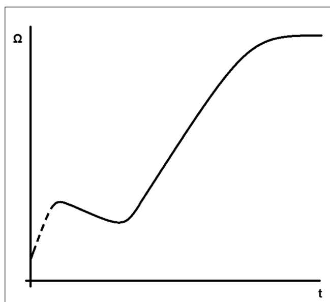
FIGURA 25. GRÁFICO DE LA RESISTENCIA DEL AISLAMIENTO
