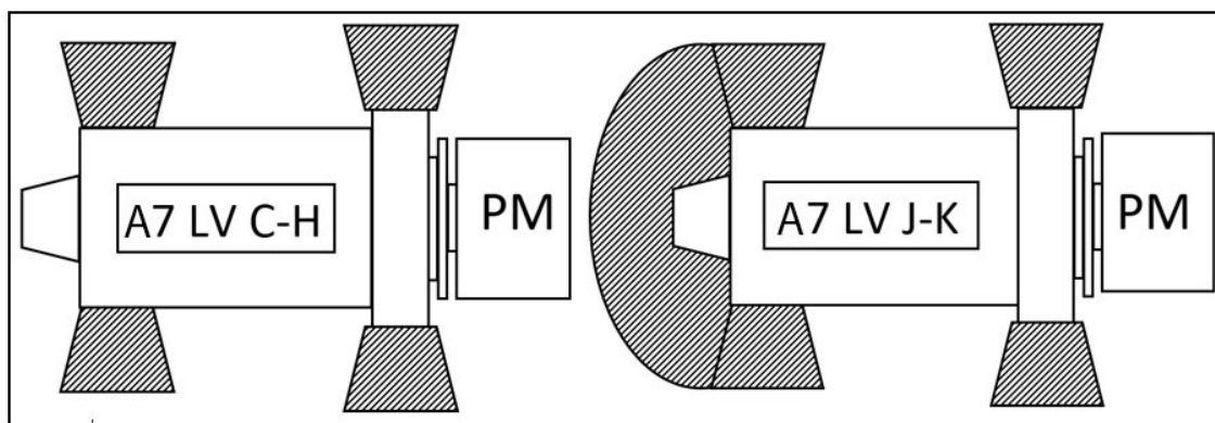
FIGURA 5. ZONAS DE PELIGRO DEL ALTERNADOR DE BAJO VOLTAJE A7
