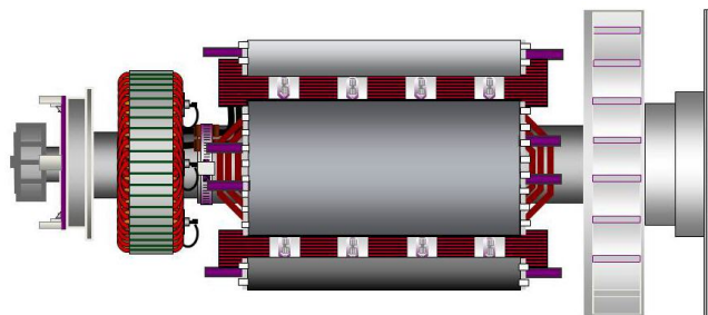
FIGURA 22. ROTOR DE ALTERNADOR DE UM ROLAMENTO COM ILUSTRAÇÃO DOS DISCOS DE ACOPLAMENTO APARAFUSADOS AO CUBO DE ACOPLAMENTO DA EXTREMIDADE MOTORA (À DIREITA)
