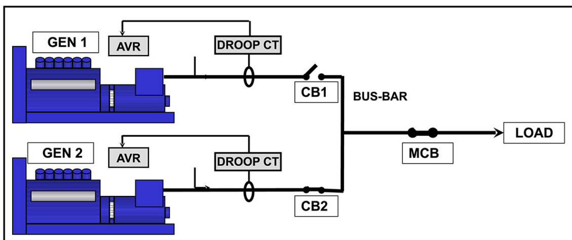
FIGURA 25. COLOCAÇÃO EM PARALELO OU SINCRONIZAÇÃO DE ALTERNADORES
