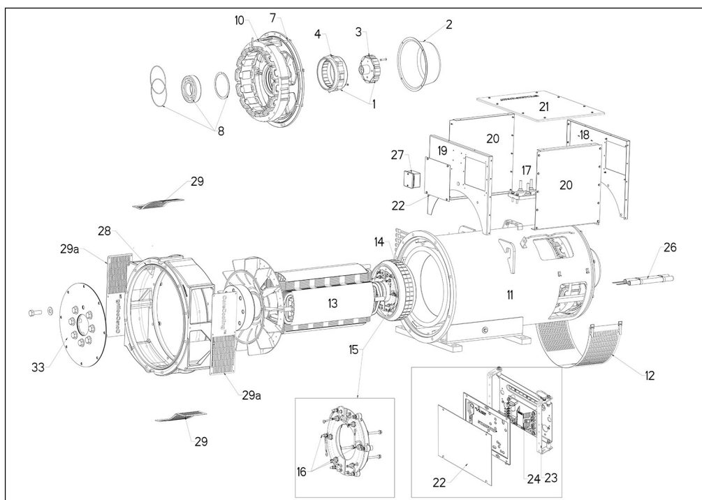
RYSUNEK 28. ALTERNATOR JEDNOŁOŻYSKOWY S4 (DEDYKOWANY)
