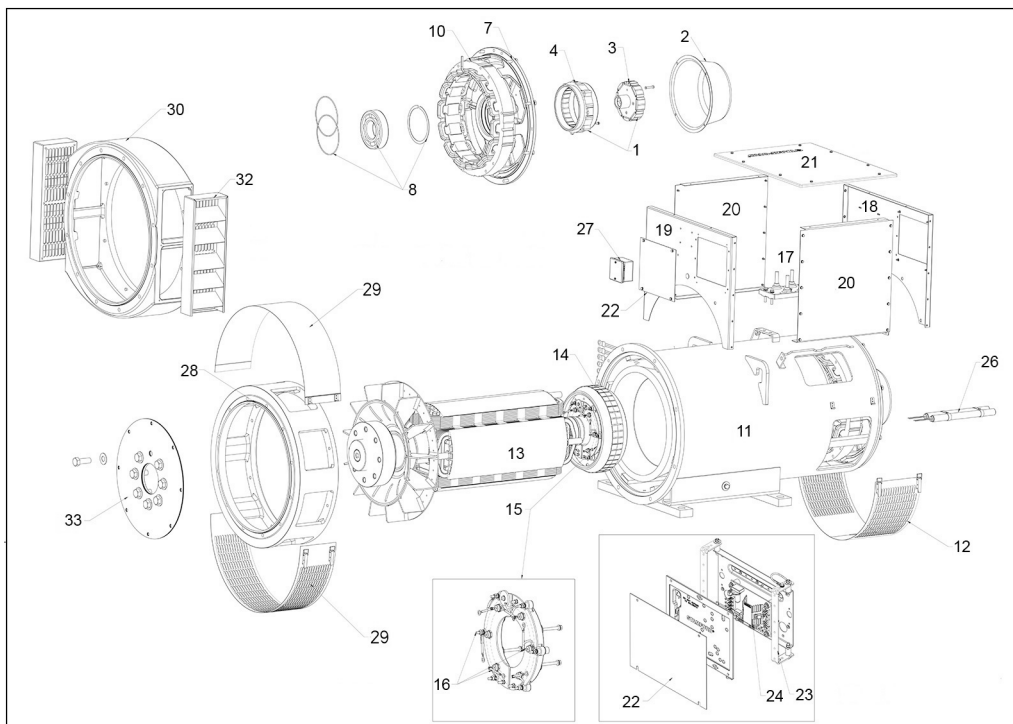
RYSUNEK 27. ALTERNATOR JEDNOŁOŻYSKOWY S4
