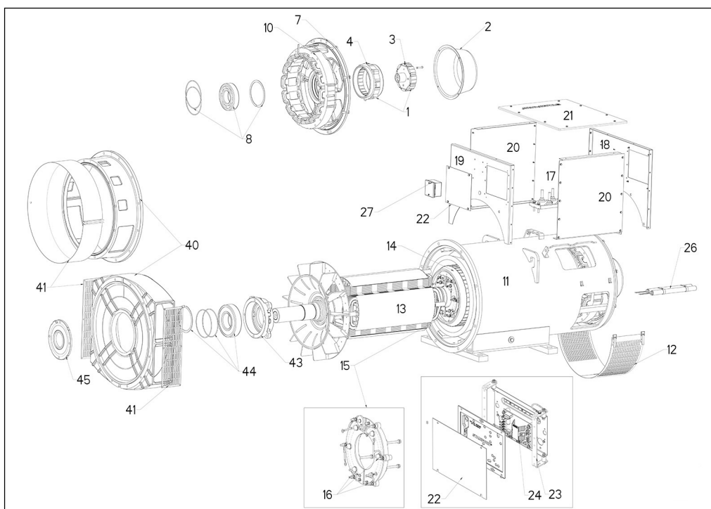
RYSUNEK 29. ALTERNATOR DWUŁOŻYSKOWY S4
