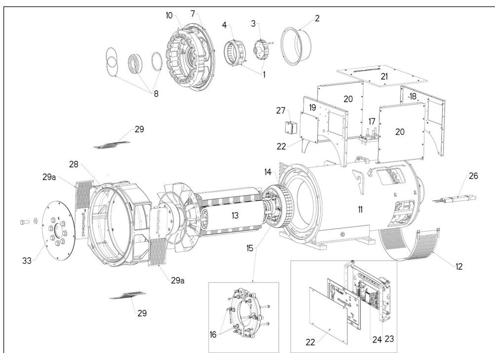
FIGURA 28. ALTERNADOR S4 COM UM ROLAMENTO (DEDICADO)
