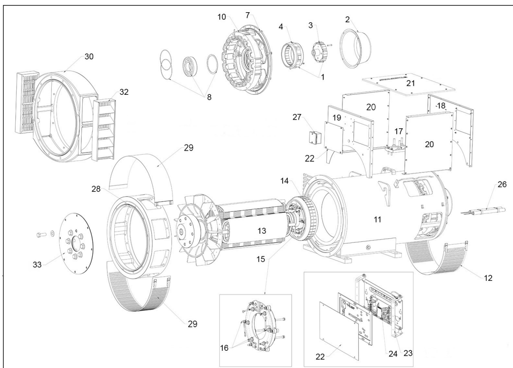
FIGURA 27. ALTERNADOR S4 COM UM ROLAMENTO
