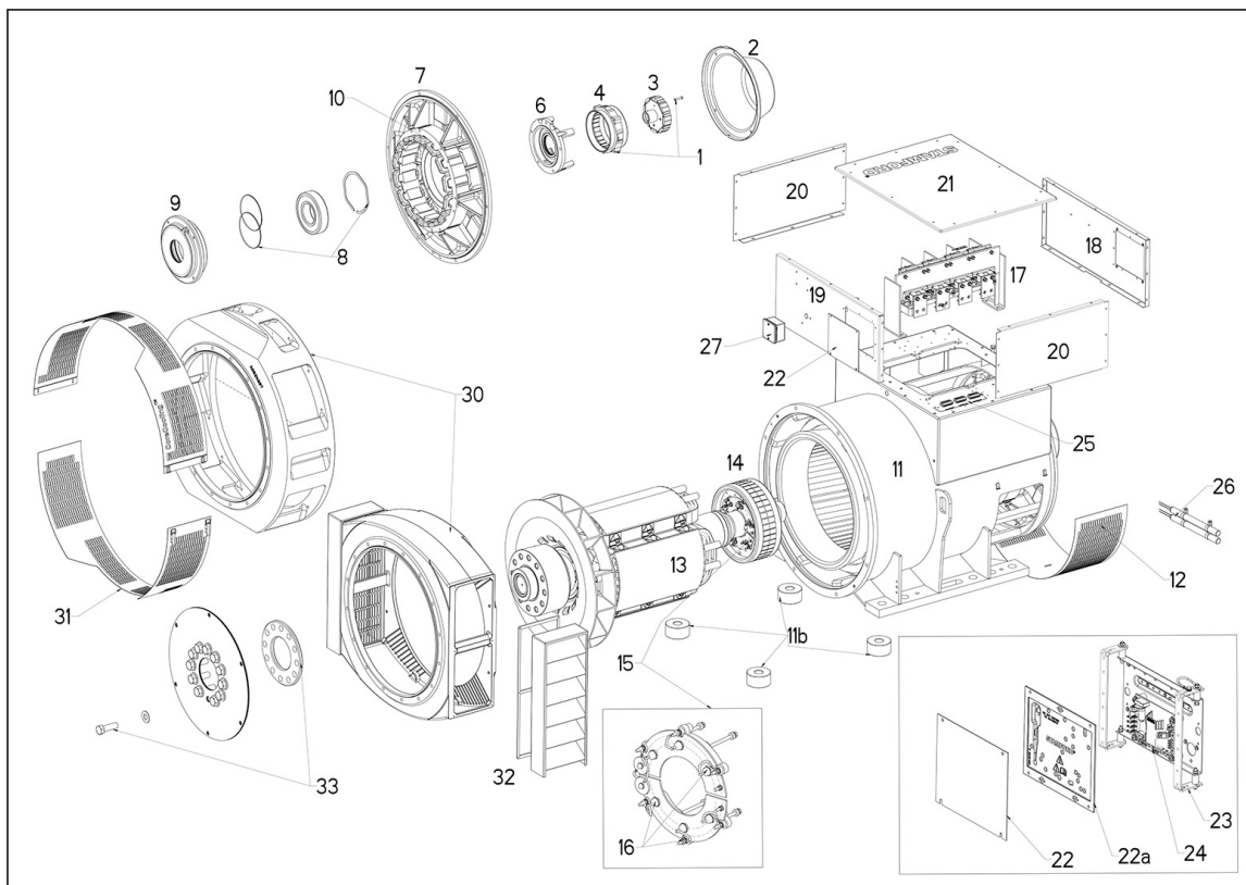
FIGURE 27. S6 - ALTERNATEUR À UN ROULEMENT - NOYAU C - F
