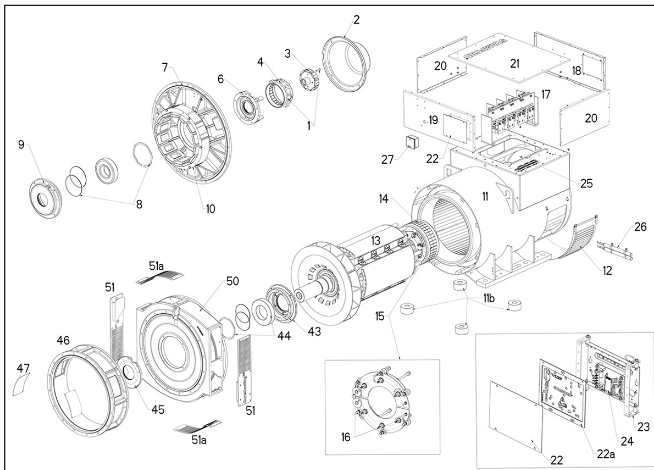
FIGURE 31. S6 - ALTERNATEUR À DEUX ROULEMENTS (DÉDIÉ) - NOYAU C - F
