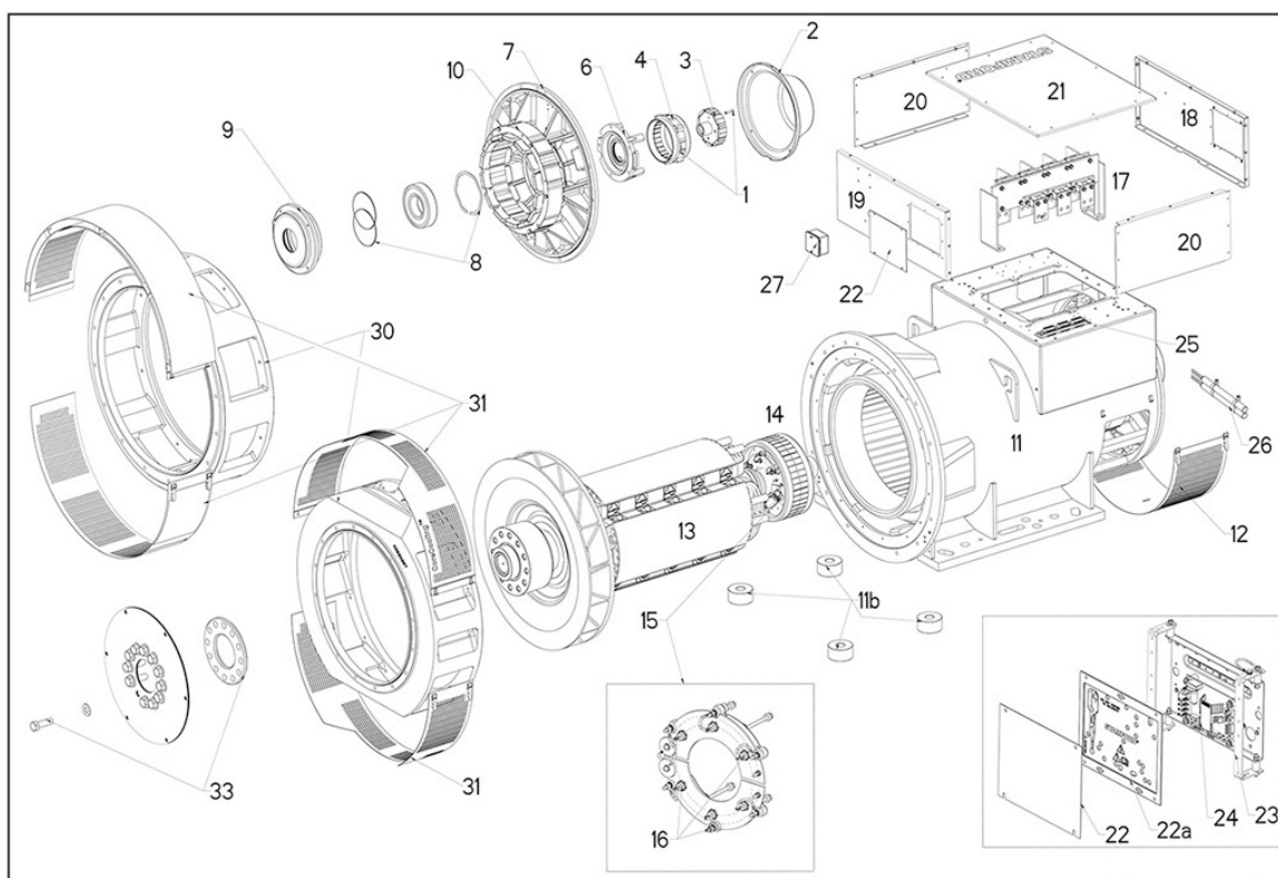
FIGURE 28. S6 - ALTERNATEUR À UN ROULEMENT - NOYAU G - H
