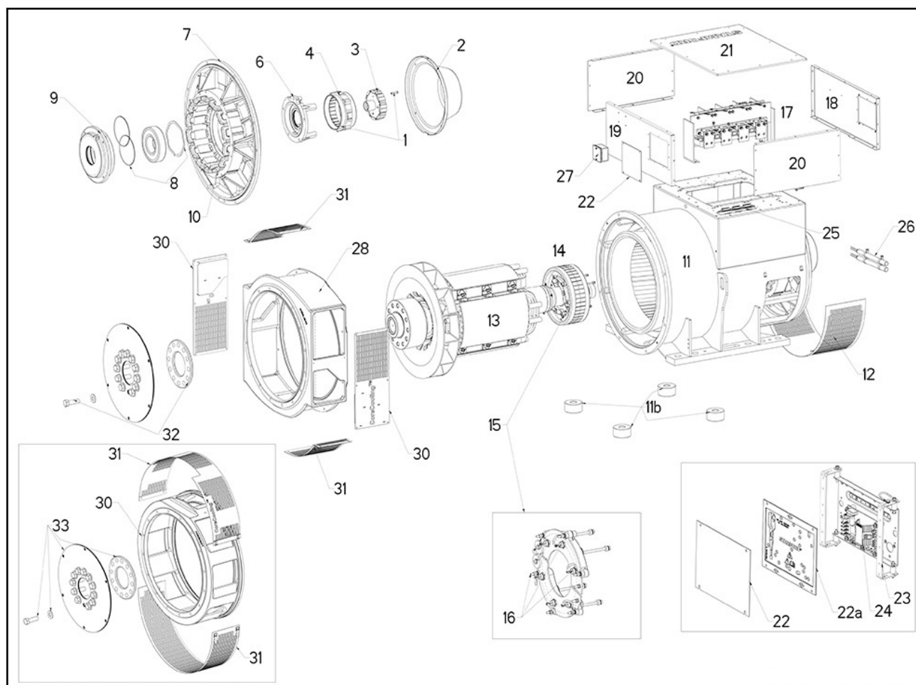
FIGURE 29. ALTERNATEUR S6 À PALIER SIMPLE (DÉDIÉ)
