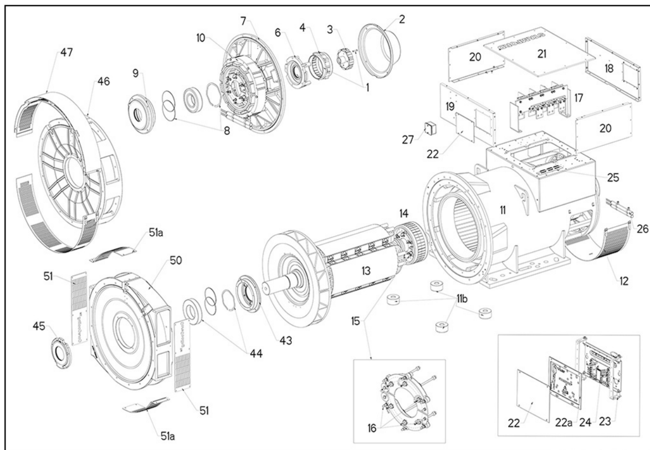
RYSUNEK 32. ALTERNATOR DWUŁOŻYSKOWY S6 (DEDYKOWANY) Z RDZENIEM G-H
