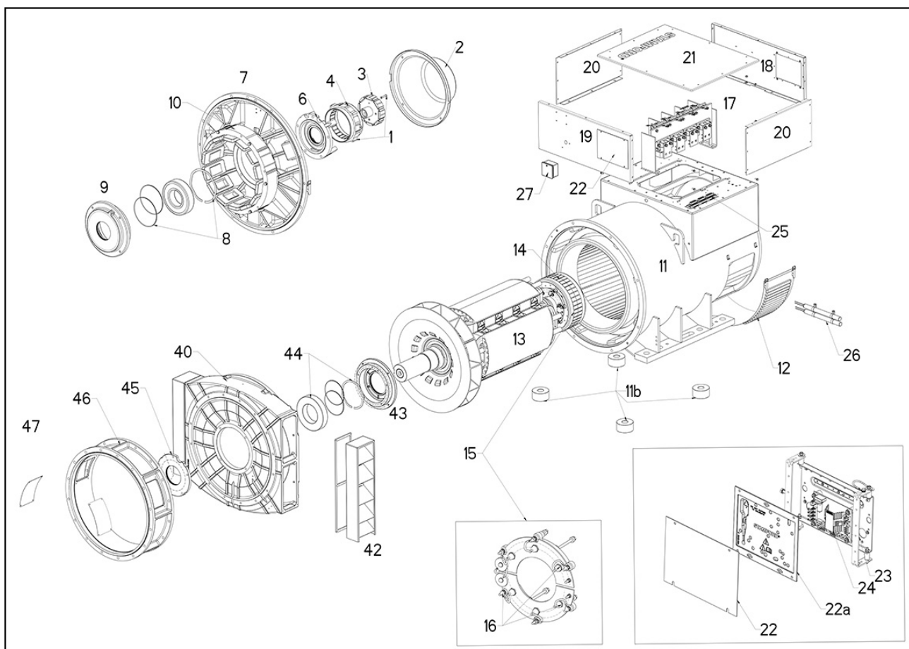
RYSUNEK 30. ALTERNATOR DWUŁOŻYSKOWY S6 Z RDZENIEM C-F
