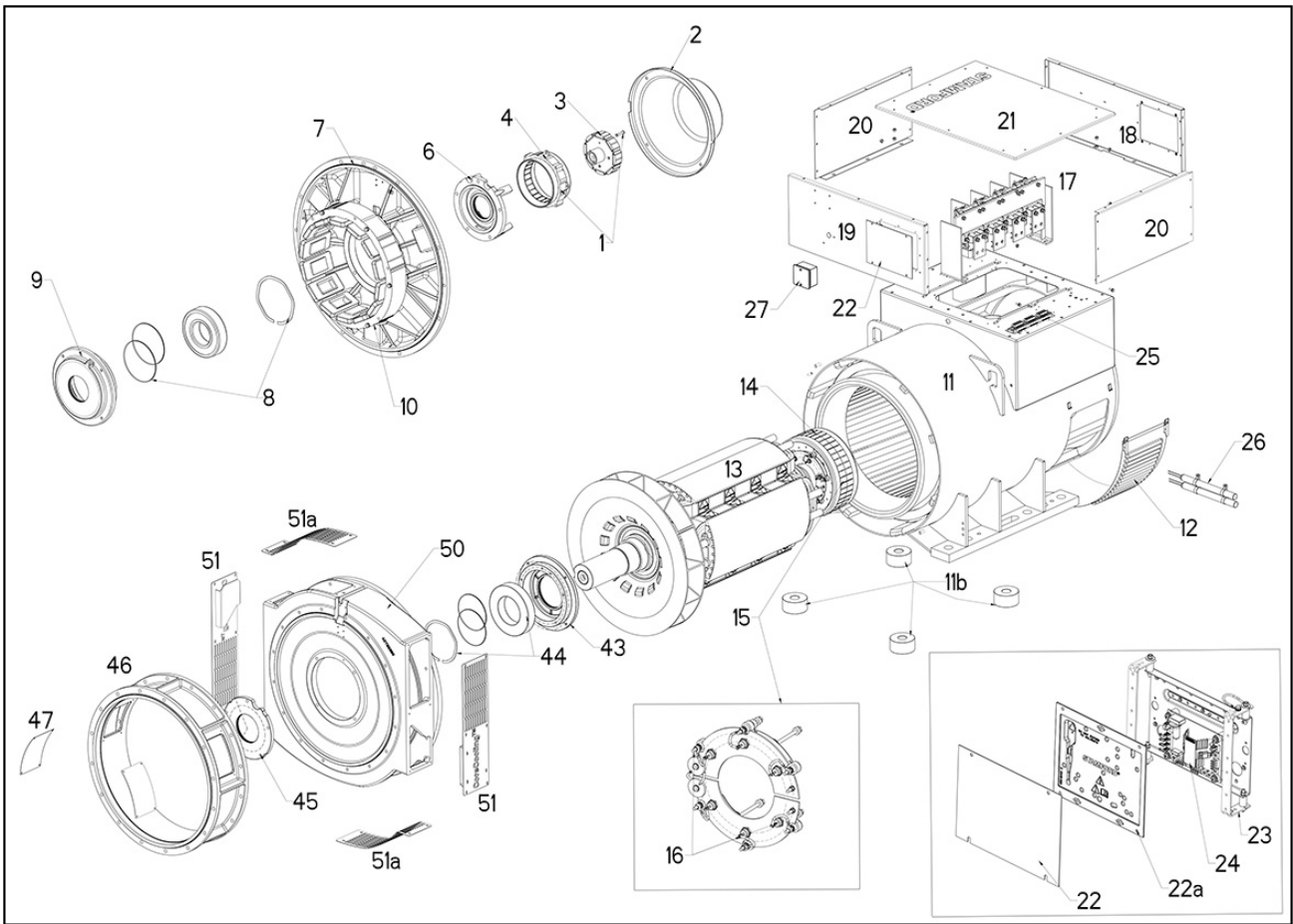
RYSUNEK 31. ALTERNATOR DWUŁOŻYSKOWY S6 (DEDYKOWANY) Z RDZENIEM C-F
