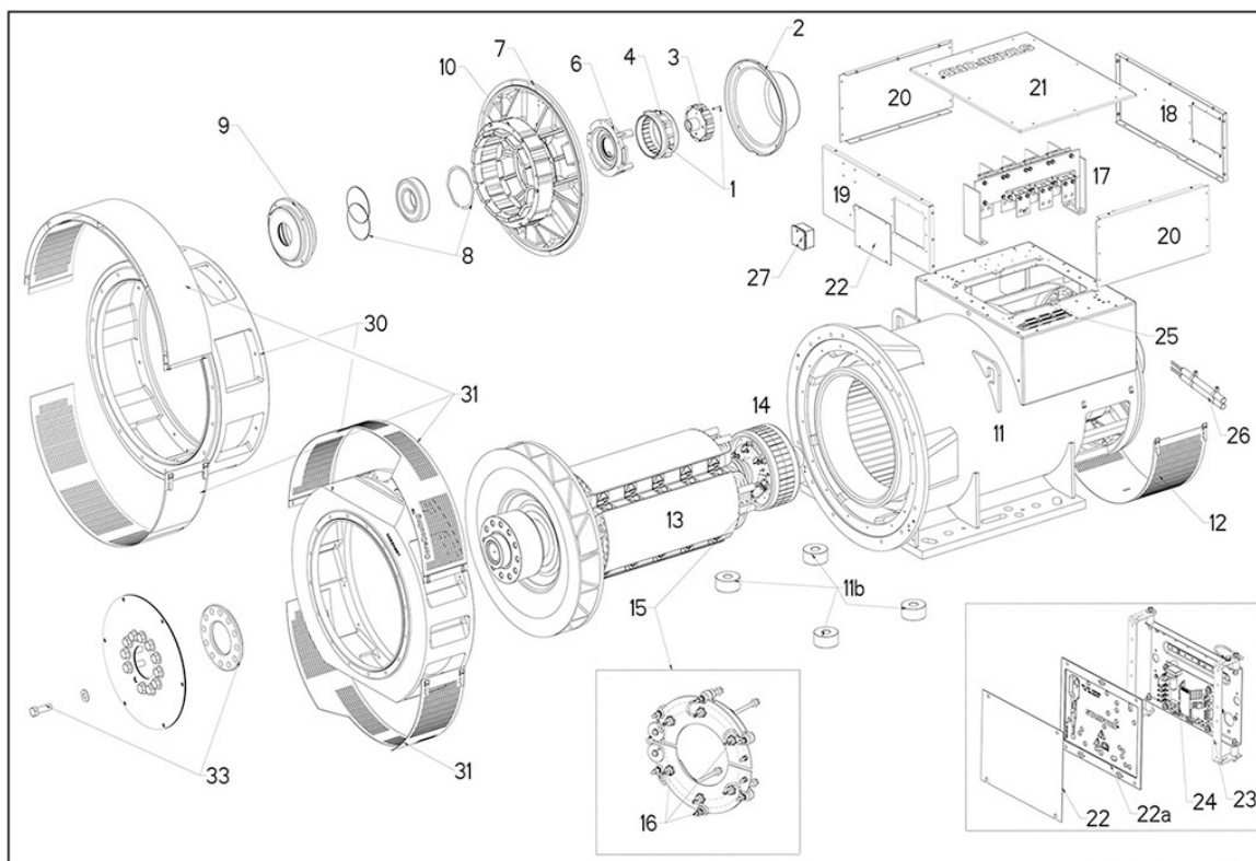
RYSUNEK 28. ALTERNATOR JEDNOŁOŻYSKOWY S6 Z RDZENIEM G-H
