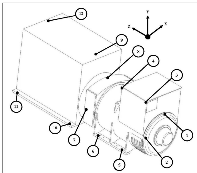
FIGURE 20. EMBLEMES DE MESURAGE DES VIBRATIONS
