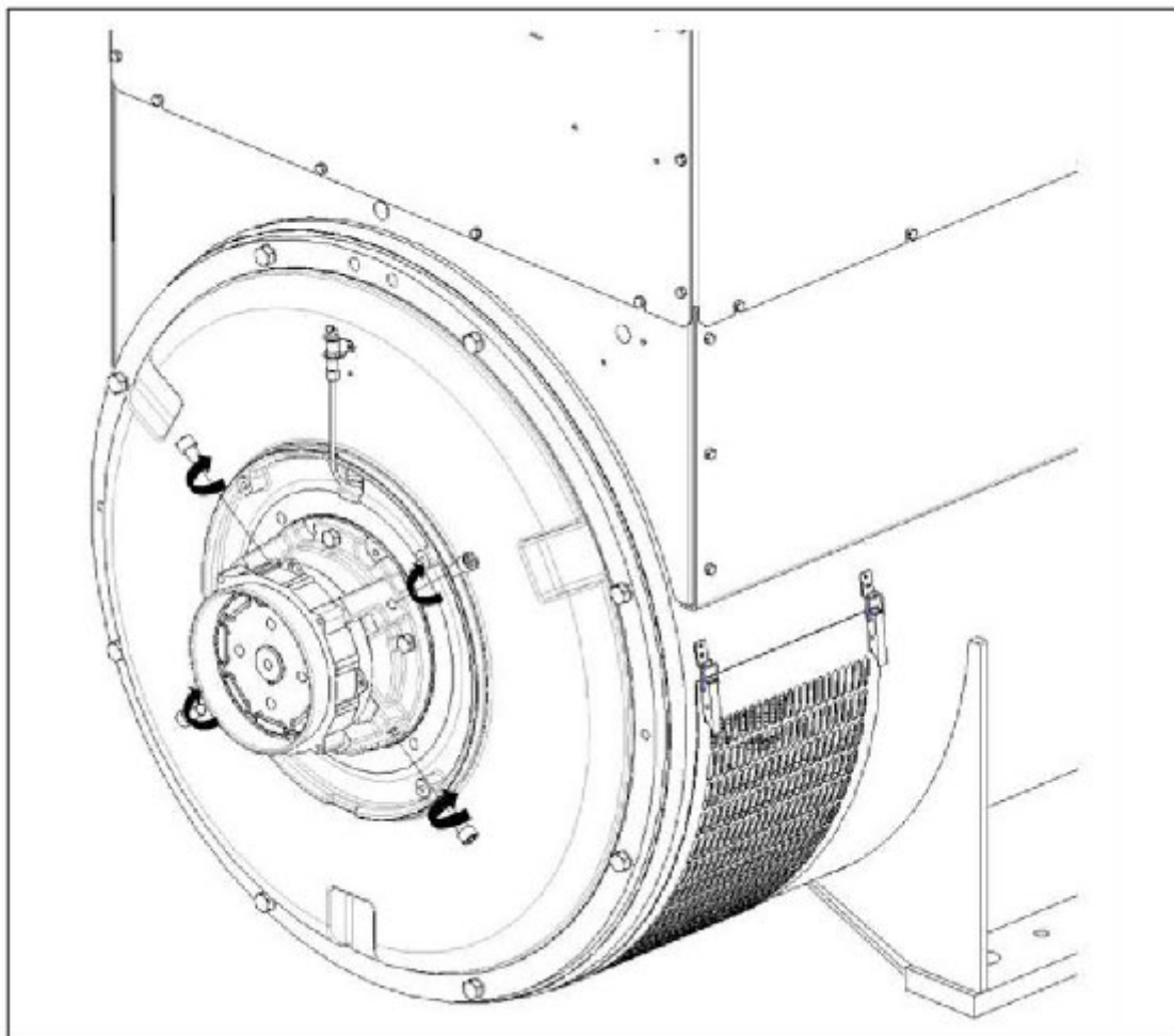
RYSUNEK 19. INSTRUKCJE WYKRĘCANIA I WKRĘCANIA ŚRUB WSPORNIKA TRANSPORTOWEGO WIRNIKA
