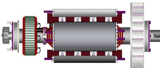
RYSUNEK 23. WIRNIK ALTERNATORA DWUŁOŻYSKOWEGO Z WIDOCZNYM WAŁEM I SZCZELINĄ NA KLUCZ UMOŻLIWIAJĄCĄ ELASTYCZNE SPRZĘGANIE (PO PRAWEJ).
