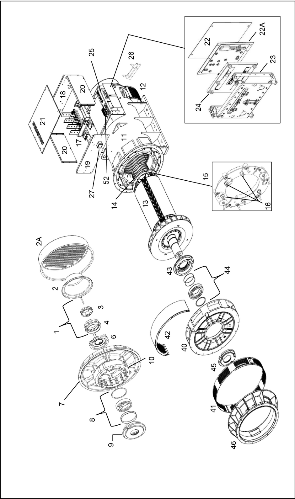
FIGURA 29. ALTERNADOR DE DOIS ROLAMENTOS S7
