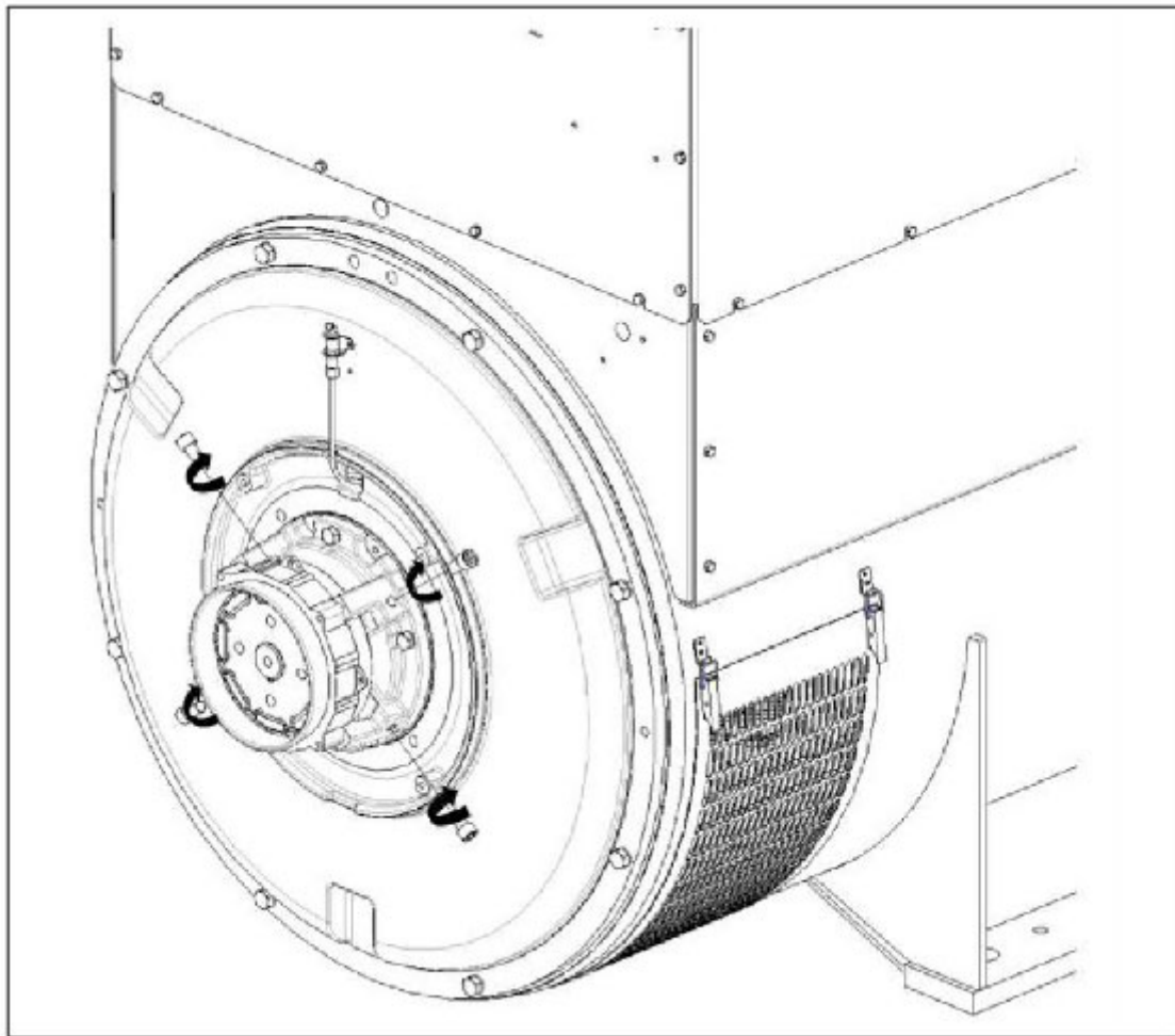
FIGURA 19. INSTRUCCIONES DE EXTRACCIÓN Y COLOCACIÓN DE LOS TORNILLOS DE SOPORTE PARA EL TRANSPORTE DEL ROTOR
