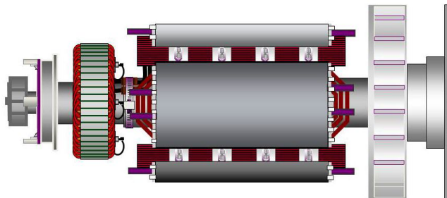
FIGURA 22. ROTOR DEL ALTERNADOR DE UN COJINETE EN EL QUE SE OBSERVAN LOS DISCOS DE ACOPLAMIENTO ATORNILLADOS AL CUBO DE ACOPLAMIENTO DEL EXTREMO IMPULSOR (A LA DERECHA)
