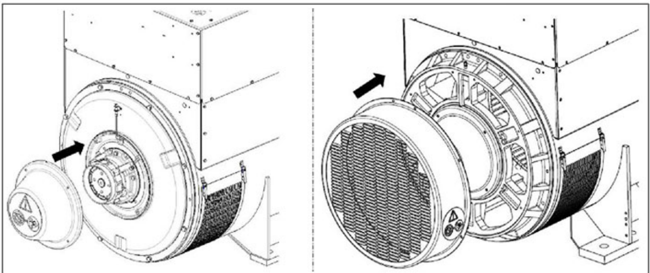
FIGURA 18. INSTRUCCIONES DE EXTRACCIÓN Y COLOCACIÓN DE LA CUBIERTA DE SOPORTE PARA EL TRANSPORTE DEL ROTOR
