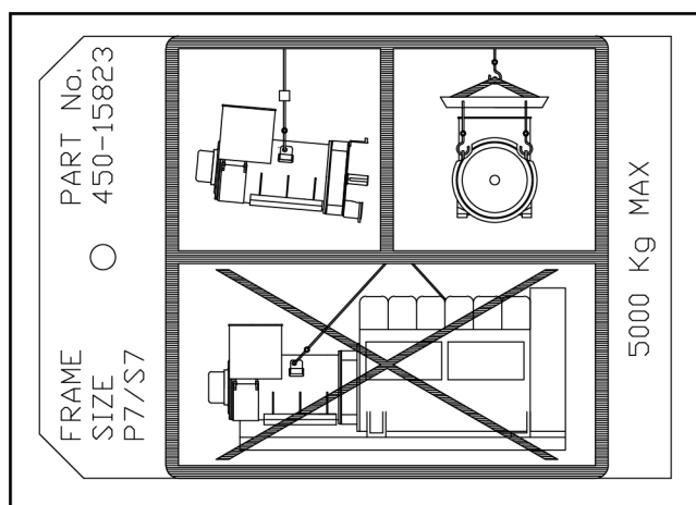
FIGURA 17. ETIQUETA DE ELEVACIÓN
