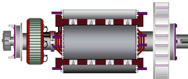
FIGUR 23. ROTORN I EN VÄXELSTRÖMSGENERATOR MED TVÅ LAGER SOM VISAR AXEL MED KILSPÅR FÖR FLEXIBEL KOPPLING (TILL HÖGER)
