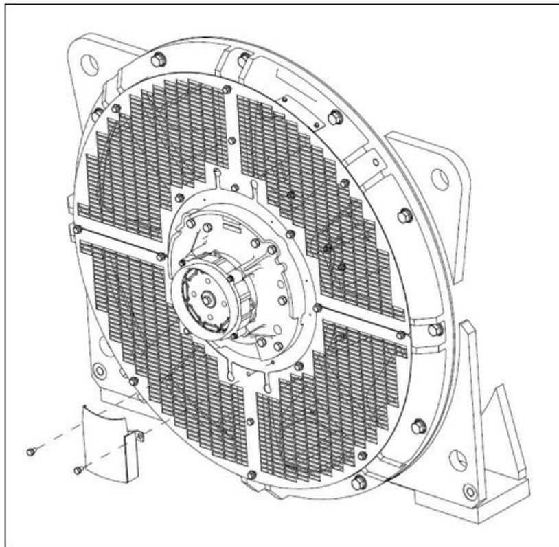
FIGURA 29. CONTENITORE DI RACCOLTA GRASSO S9
