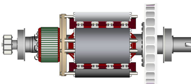
FIGURA 23. ROTORE DELL'ALTERNATORE A DUE CUSCINETTI CON ALBERO CON CHIAVETTA PER ACCOPPIAMENTO FLESSIBILE (A DESTRA)
