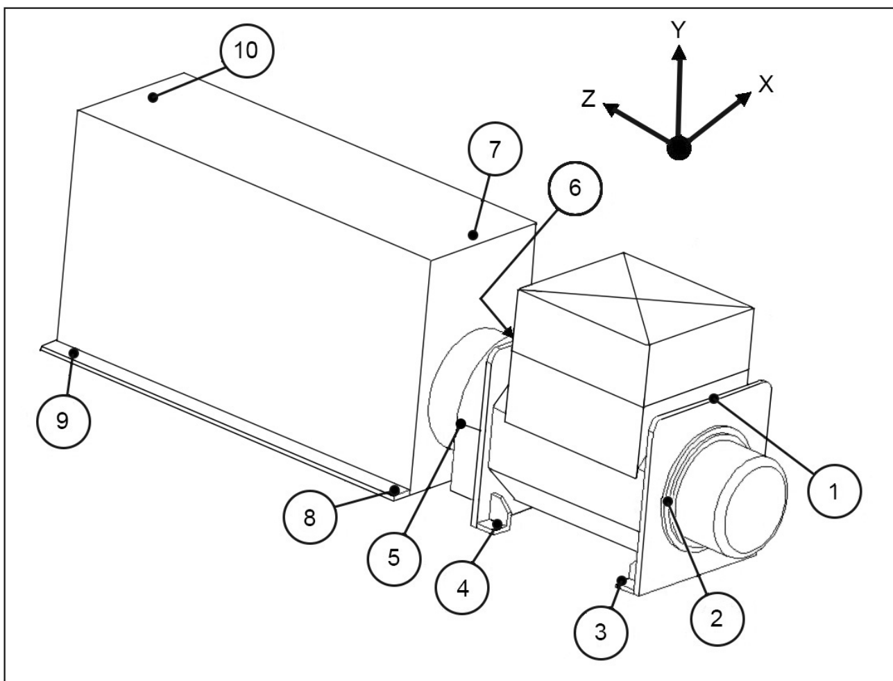
FIGURA 20. PUNTI DI MISURAZIONE DELLE VIBRAZIONI
