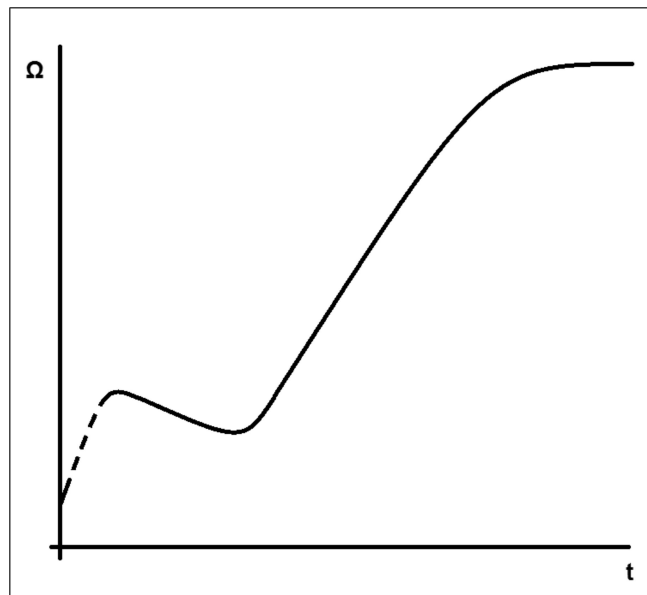
FIGURA 31. GRAFICO RESISTENZA DI ISOLAMENTO
