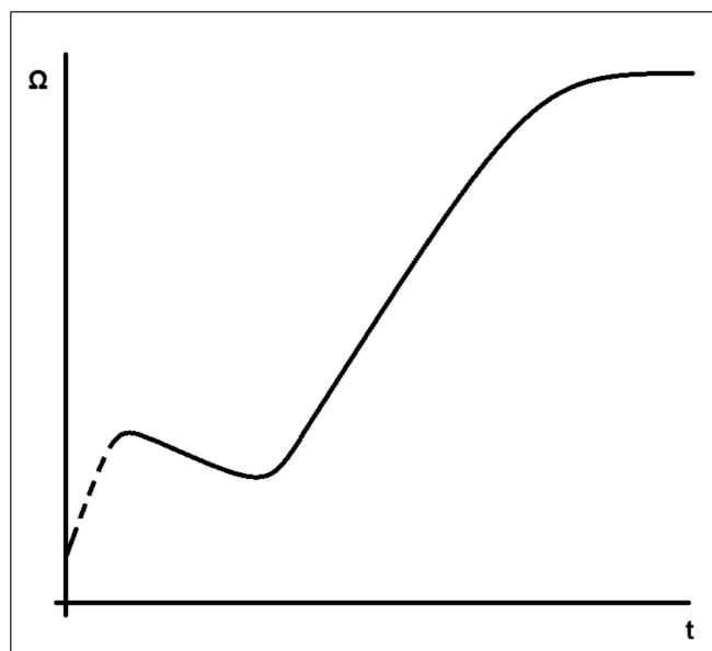
図 31. 絶縁抵抗のグラフ
