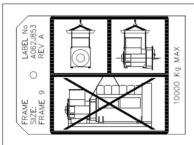
図 17. リフティング ラベルの例
