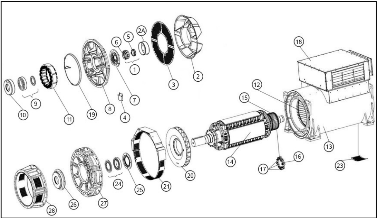
図 33. S9 低電圧 2 ベアリング オルタネーター
