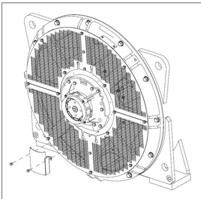
図 29. グリーストラップ S9
