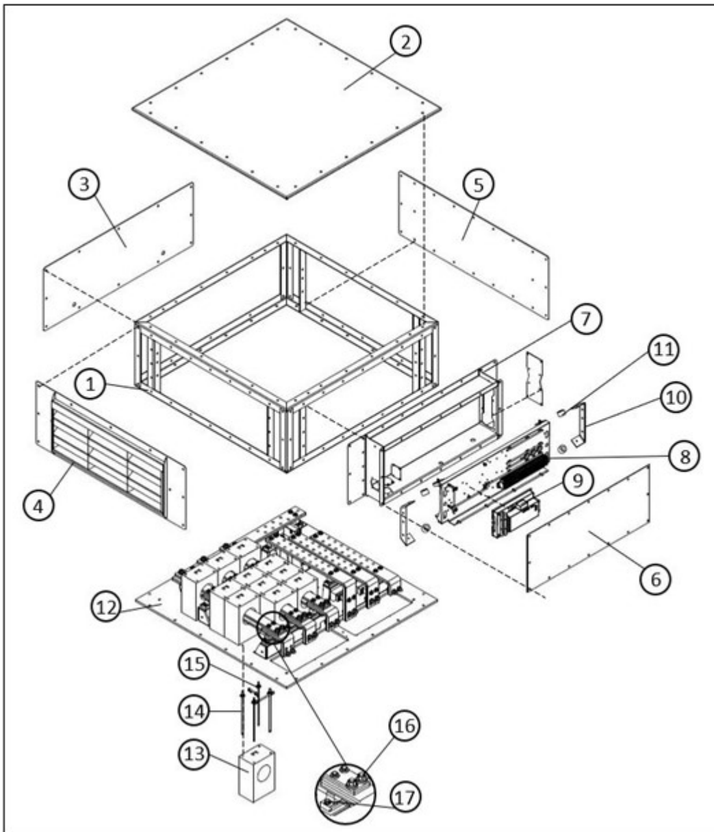
図 34. S9 低圧端子ボックス
