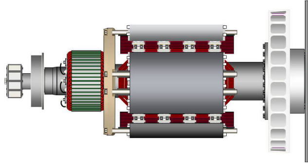
図 22. ドライブ エンド カップリング ハブにボルトで固定されたカップリング ディスクを示すベアリング オルタネーター ローター (右)
