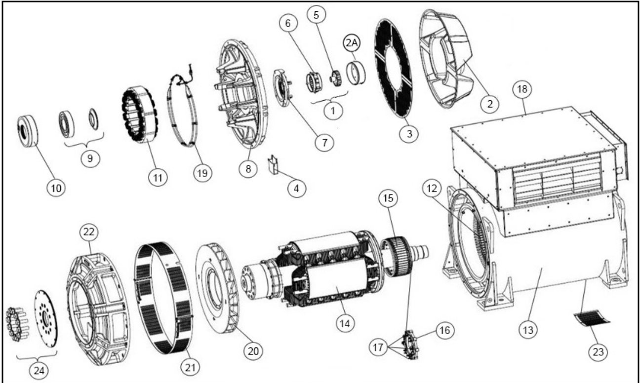
図 32. S9 低電圧 1 ベアリング オルタネーター
