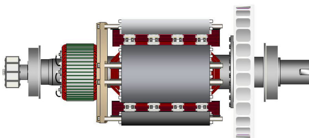
FIGURA 23. ROTOR DE ALTERNADOR DE DOIS ROLAMENTOS COM ILUSTRAÇÃO DO VEIO COM ESCATEL PARA ACOPLAMENTO FLEXÍVEL (À DIREITA)
