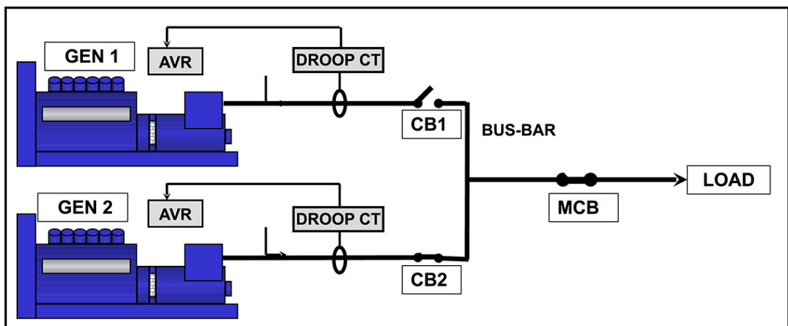
FIGURA 28. COLOCAÇÃO EM PARALELO OU SINCRONIZAÇÃO DE ALTERNADORES
