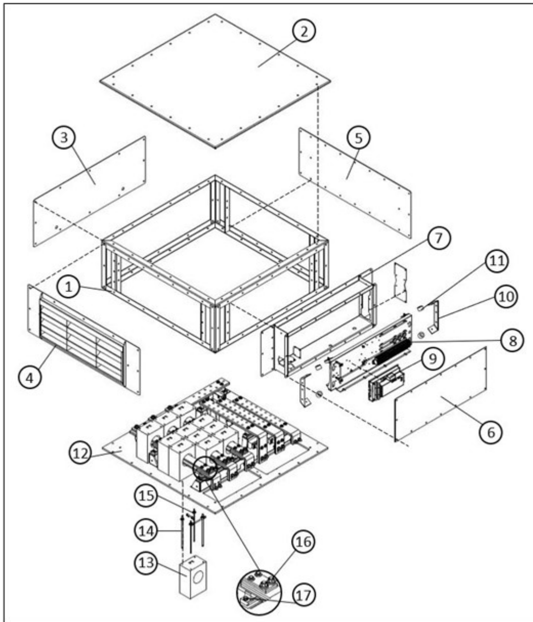
FIGURA 34. CAIXA DE TERMINAIS S9 DE BAIXA TENSÃO
