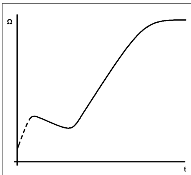
FIGURA 31. GRÁFICO DE RESISTÊNCIA DE ISOLAMENTO
