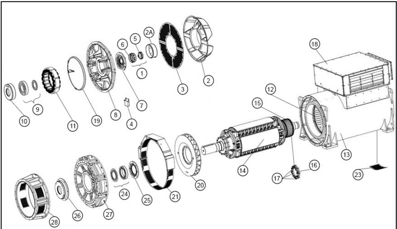
FIGURA 33. ALTERNADOR DE DOIS ROLAMENTOS S9 DE BAIXA TENSÃO
