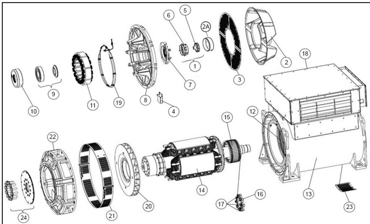
FIGURA 32. ALTERNADOR S9 DE BAJO VOLTAJE DE UN COJINETE
