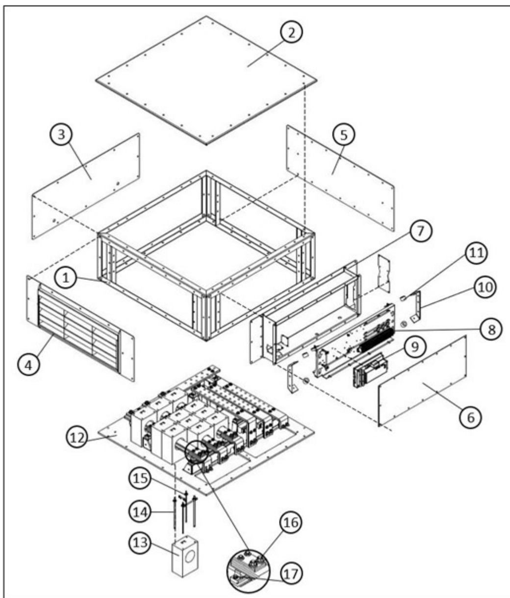
FIGURA 34. CAJA DE BORNES DE S9 DE BAJO VOLTAJE
