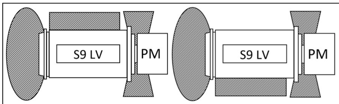
FIGURA 5. ZONAS DE PELIGRO DEL ALTERNADOR DE BAJO VOLTAJE S9
