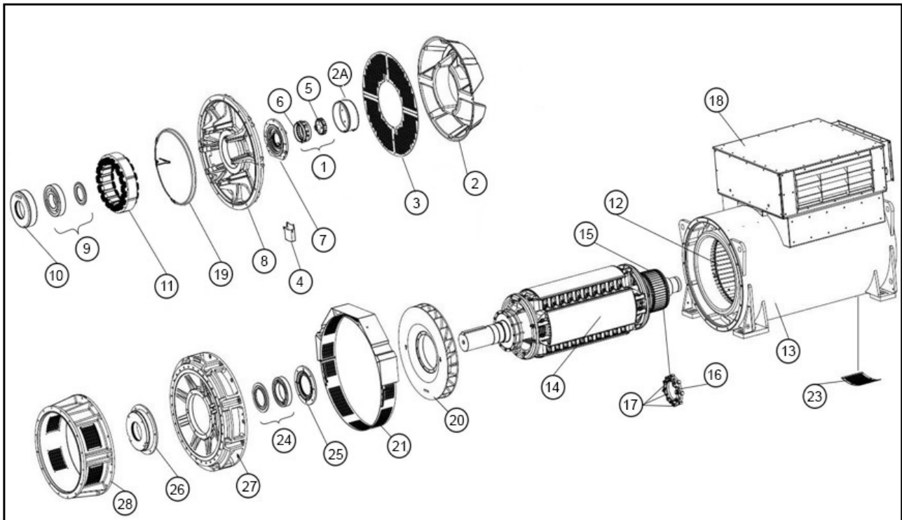
FIGURA 33. ALTERNADOR S9 DE BAJO VOLTAJE DE DOS COJINETES
