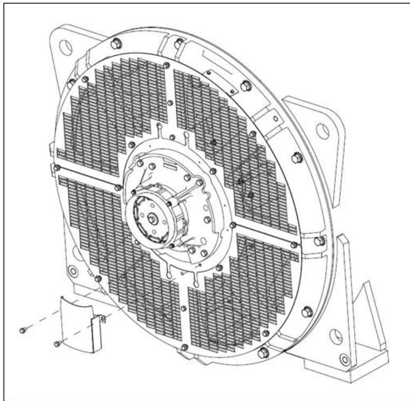
FIGURA 29. TRAMPA DE GRASA DE S9
