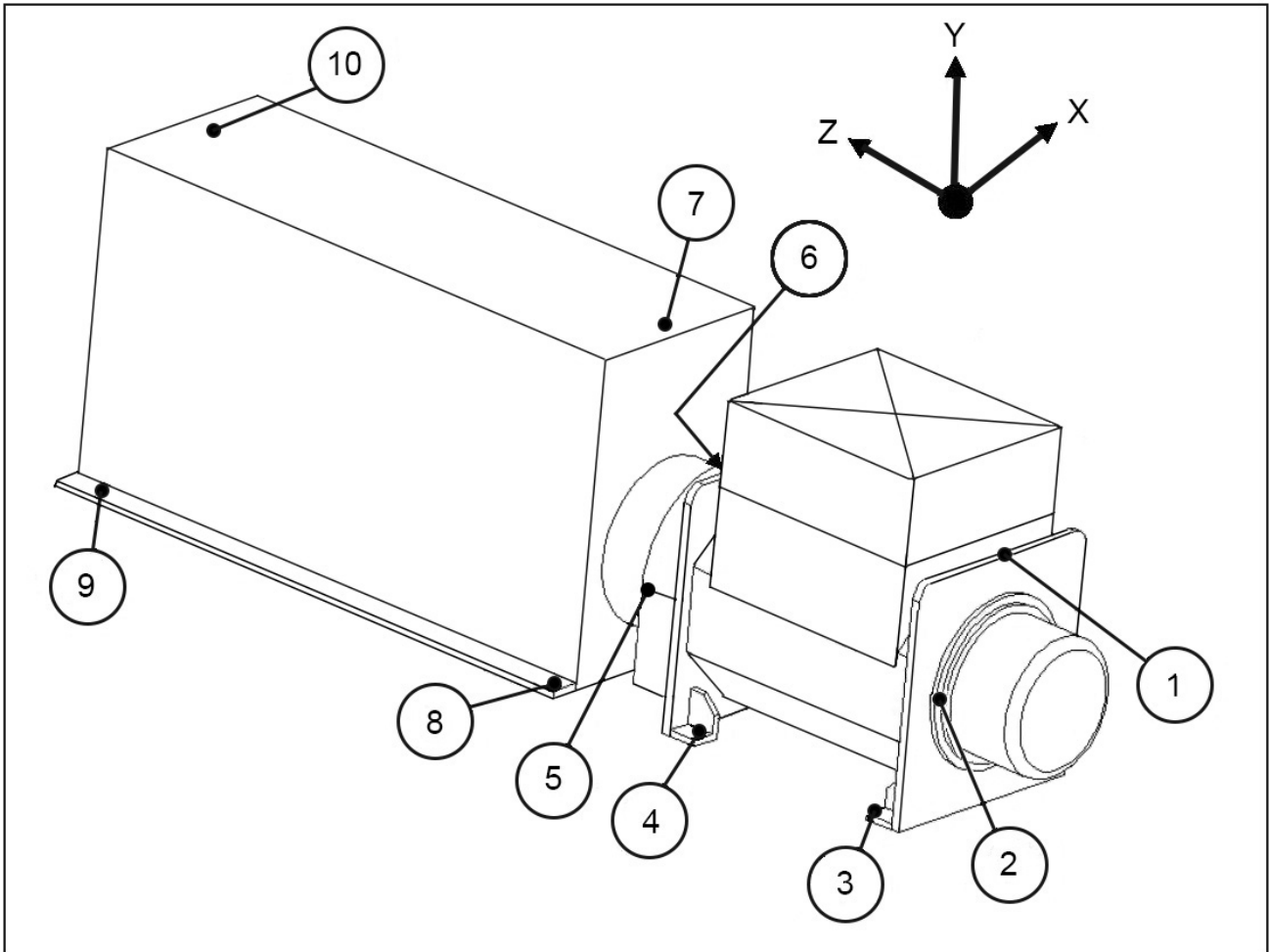
FIGURA 20. POSICIONES DE MEDICIÓN DE LA VIBRACIÓN
