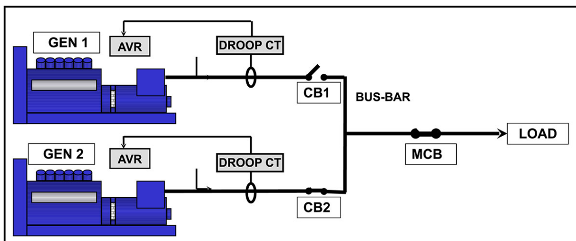
FIGURA 28. ALTERNADORES PARALELOS O DE SINCRONIZACIÓN
