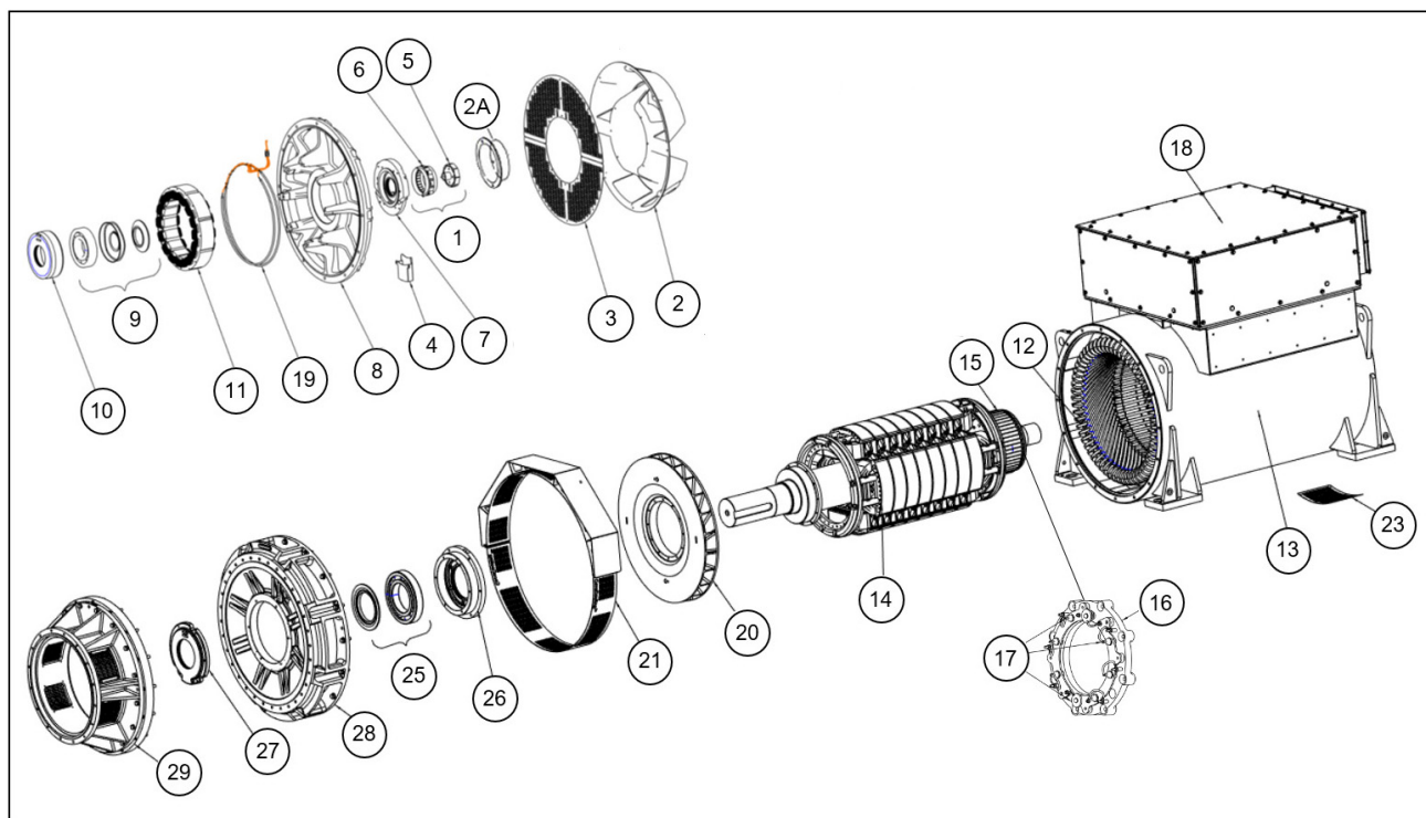
FIGURA 29. ALTERNADOR DE DOIS ROLAMENTOS S9
