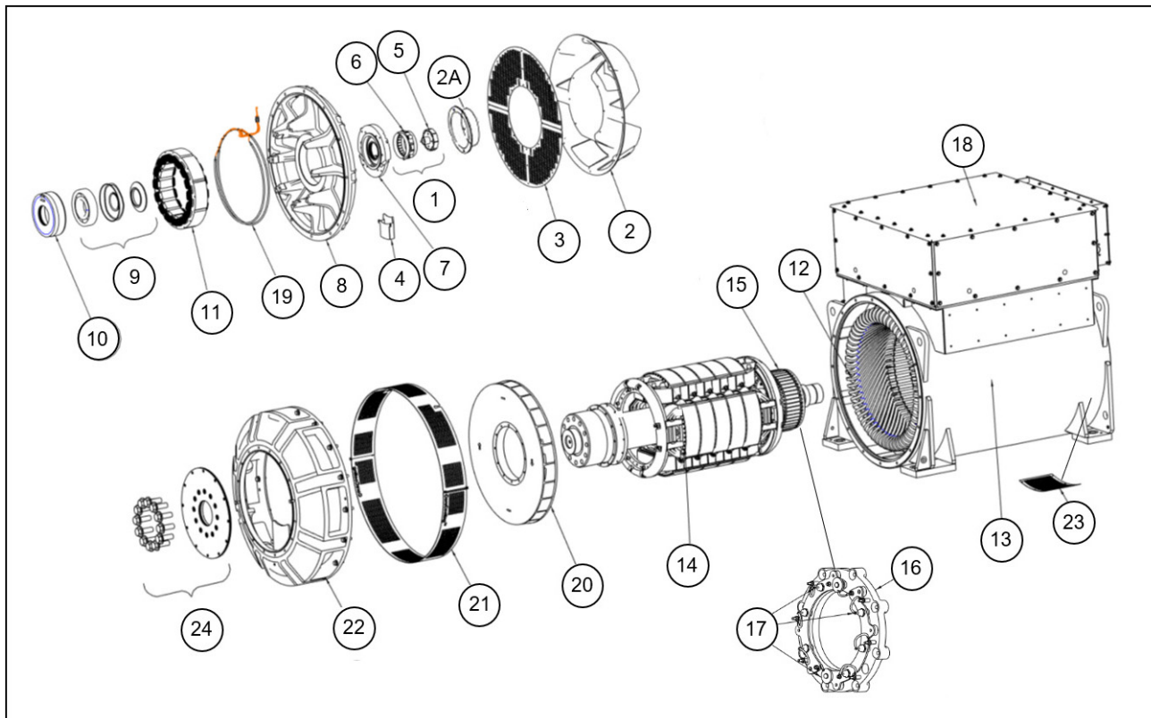
FIGURA 28. ALTERNADOR S9 COM UM ROLAMENTO
