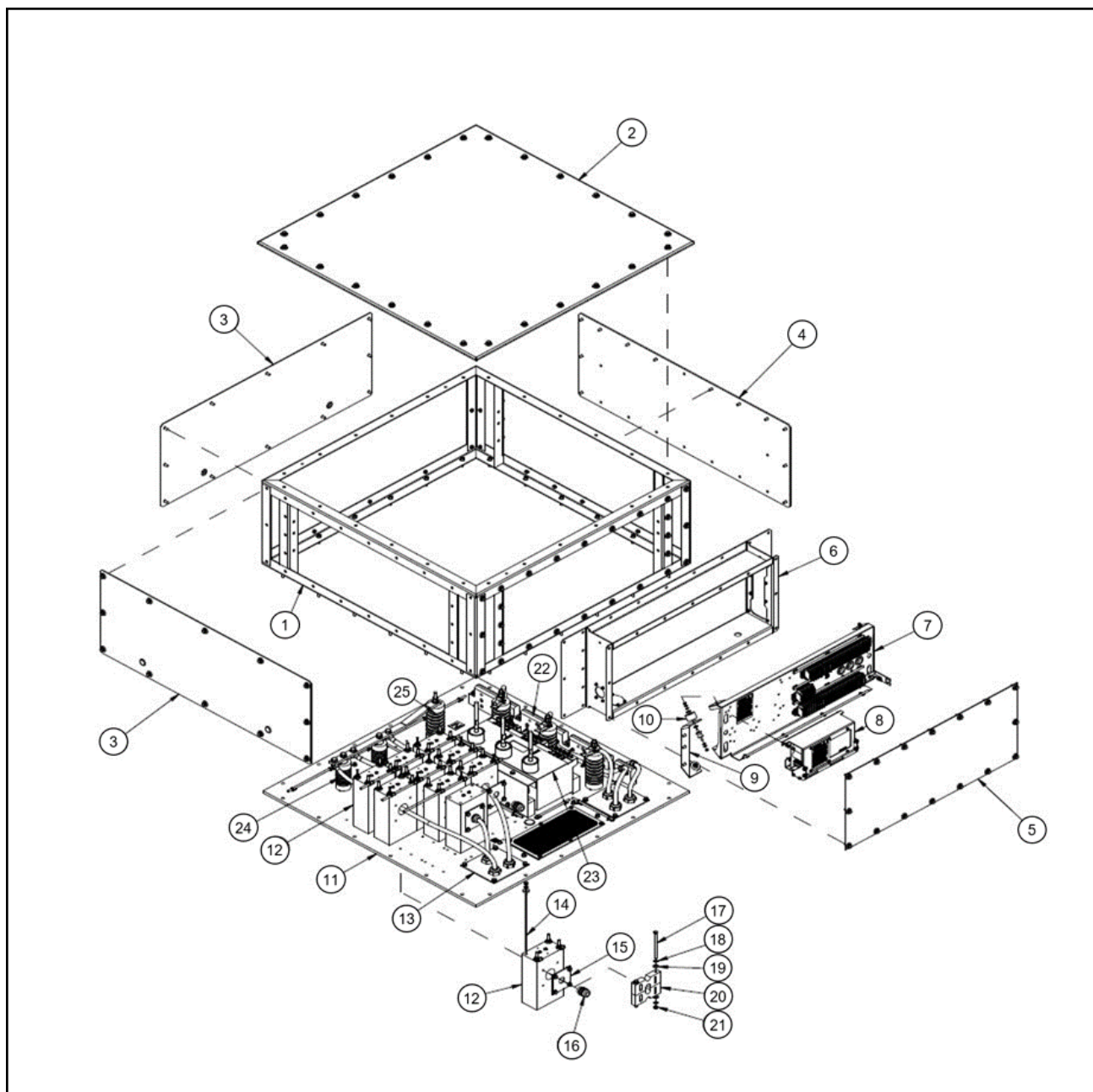
FIGURA 30. PEÇAS E FIXADORES DA CAIXA DE TERMINAIS DE MÉDIA E ALTA TENSÃO
