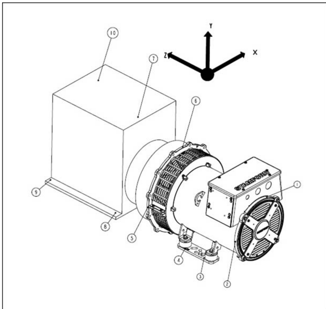
FIGURE 18. POSITIONS DE MESURAGE DES VIBRATIONS
