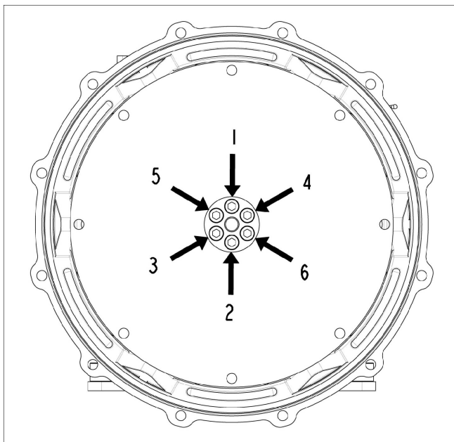
RYSUNEK 22. KOLEJNOŚĆ MOCOWANIA NA PIAŚCIE
