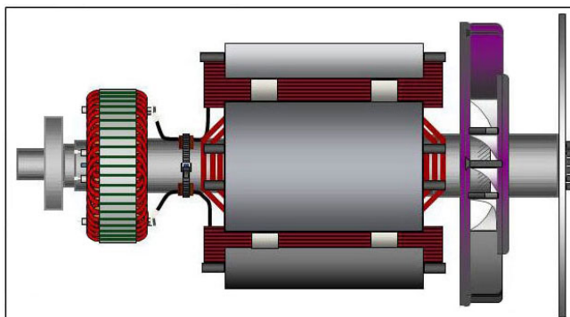
RYSUNEK 20. ALTERNATOR JEDNOŁOŻYSKOWY Z WIDOCZNYMI TARCZAMI SPRZĘGŁA PRZYKRĘCONYMI DO PIASTY SPRZĘGŁA PO STRONIE NAPEĐDOWEJ (PO PRAWEJ STRONIE)
