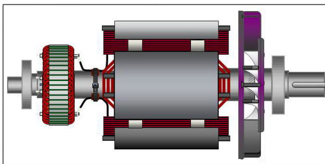
RYSUNEK 21. WIRNIK ALTERNATORA DWULOŻYSKOWEGO Z WIDOCZNYM WAŁEM I SZCELINĄ NA KLUCZ UMOŻLIWIAJĄCĄ ELASTYCZNE SPRZĘGANIE (PO PRAWEJ).
