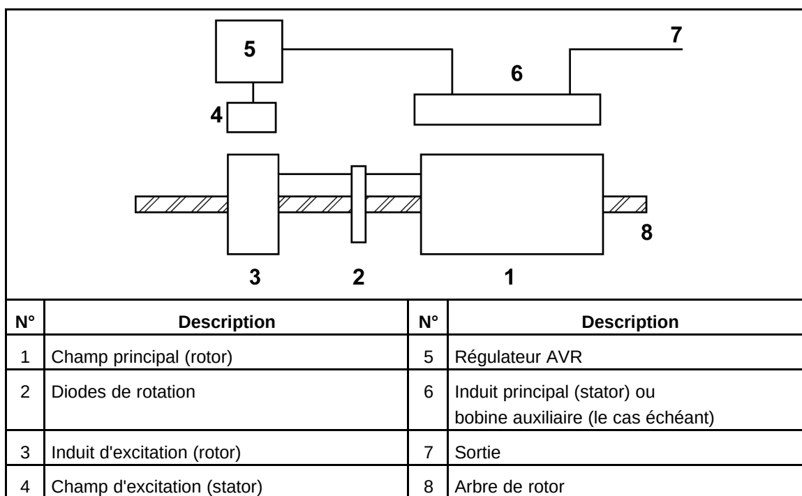
TABEAU 2. PRINCIPAUX RÉGULATEURS AVR ALIMENTÉS PAR STATOR
