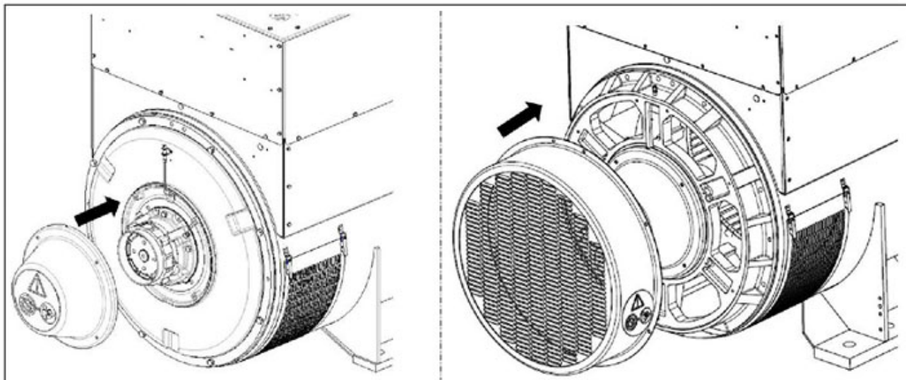
FIGURE 18. INSTRUCTIONS DE DÉPOSE ET DE MONTAGE DU COUVERCLE DU SUPPORT DE TRANSIT DU ROTOR
