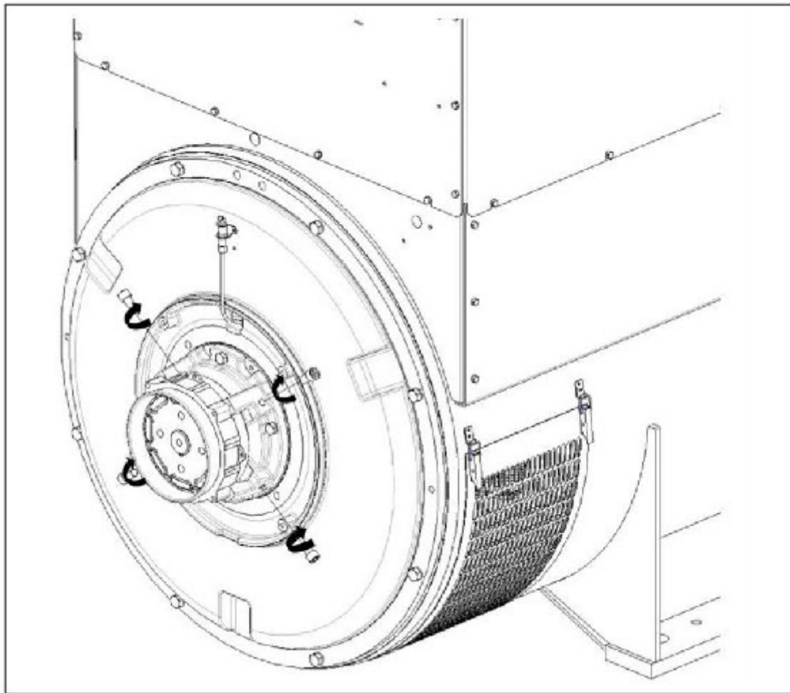
FIGURE 19. VIS DE SUPPORT DE TRANSIT DU ROTOR - INSTRUCTIONS DE DÉPOSE ET DE MONTAGE
