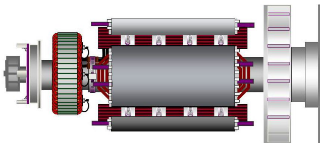
FIGURE 22. UN ROTOR D'ALTERNATEUR À ROULEMENT MONTRANT DES DISQUES D'ACCOUPLEMENT BOULONNÉS AU MOYEU D'ACCOUPLEMENT DE L'EXTRÉMITÉ D'ENTRAÎNEMENT (CÔTÉ DROIT)
