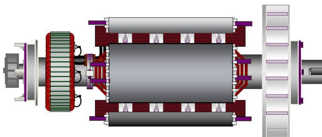
FIGURE 23. ROTOR D'ALTERNATEUR À DEUX ROULEMENTS MONTRANT UN ARBRE AVEC RAINURE POUR ACCOUPLEMENT FLEXIBLE (CÔTÉ DROIT)
