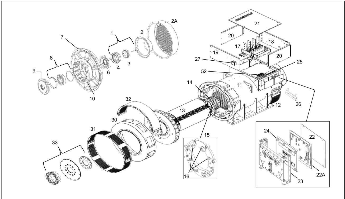
ABBILDUNG 28. S7 EINLAGER-GENERATOR
