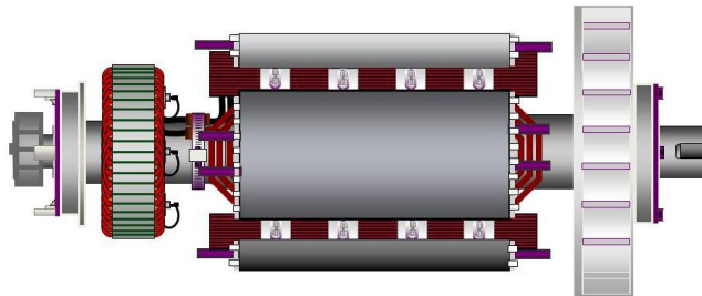
ABBILDUNG 23. ZWEILAGER-GENERATORROTOR MIT WELLE UND KEILNUT FÜR DIE ELASTISCHE KUPPLUNG (RECHTS)
