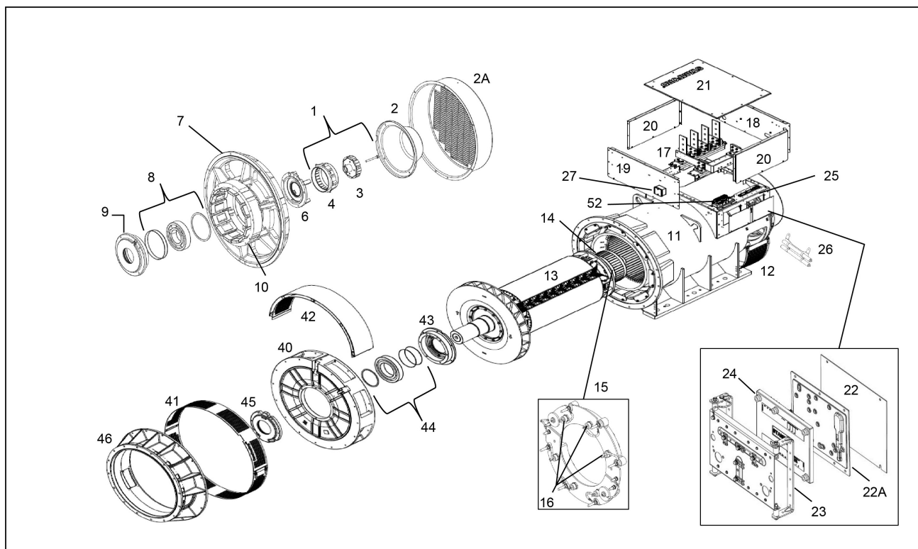
FIGURA 29. ALTERNADOR DE DOIS ROLAMENTOS S7
