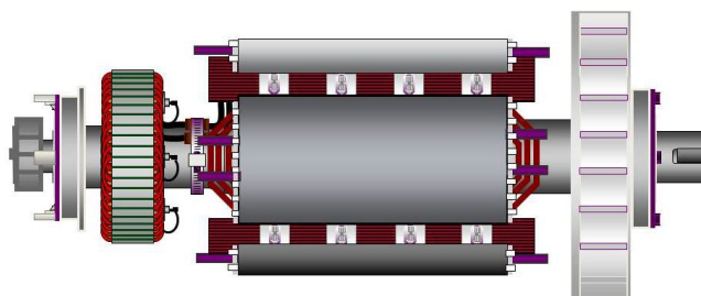
FIGURA 23. ROTOR DE ALTERNADOR DE DOIS ROLAMENTOS COM ILUSTRAÇÃO DO VEIO COM ESCATEL PARA ACOPLAMENTO FLEXÍVEL (LADO DIREITO)
