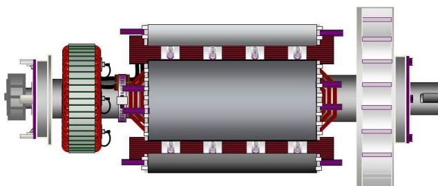
FIGURA 23. ROTOR DE ALTERNADOR CON DOS COJINETES, EN EL QUE SE APRECIA EL EJE CON CHAVETERO PARA EL ACOPLAMIENTO FLEXIBLE (LADO DERECHO)
