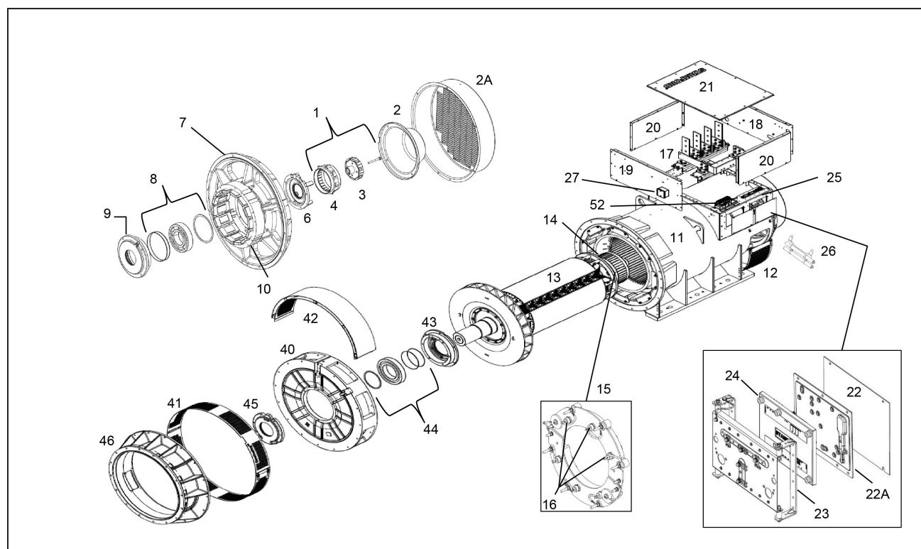
FIGURA 29. ALTERNADOR DE DOS COJINETES S7
