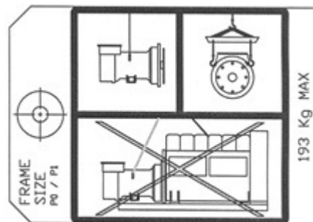
RYSUNEK 4. ETYKIETA PRZEDSTAWIAJĄCA SPOSÓB PODNOSZENIA ALTERNATORA
