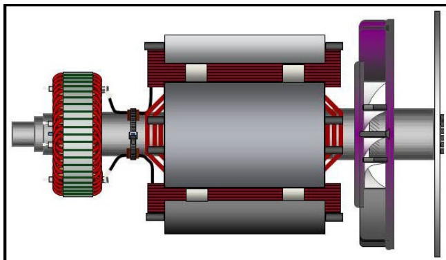
RYSUNEK 5. WIRNIK ALTERNATORA JEDNOŁOŻYSKOWEGO Z WIDOCZNYMI TARCZAMI SPRZĘGŁA SKRĘCONYMI Z PIASTĄ CZĘŚCI NAPĘDOWEJ (PO PRAWEJ).
