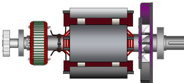
RYSUNEK 6. WIRNIK ALTERNATORA DWUŁOŻYSKOWEGO Z WIDOCZNYM WAŁEM I SZCZELINĄ NA KLUCZ UMOŻLIWIAJĄCĄ ELASTYCZNE SPRZĘGANIE (PO PRAWEJ).
