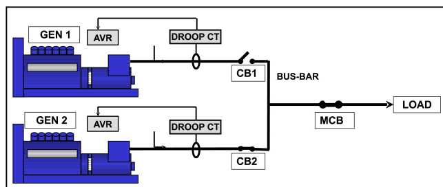
图 23. 并联或同步交流发电机
