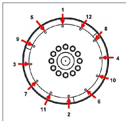
FIGURE 22. SÉQUENCE FIXE
