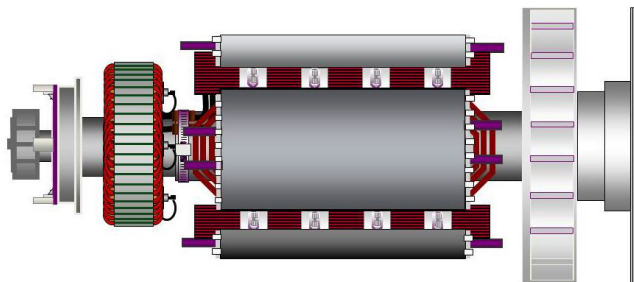
FIGURE 20. ROTOR D'ALTERNATEUR À UN PALIER MONTRANT LES DISQUES D'ACCOUPLEMENT BOULONNÉS AU MOYEU D'ACCOUPLEMENT DE L'EXTREMITÉ MOTRICE (À DROITE)
