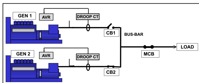
FIGURA 23. ALTERNATORI IN PARALLELO O A SINCRONIZZAZIONE
