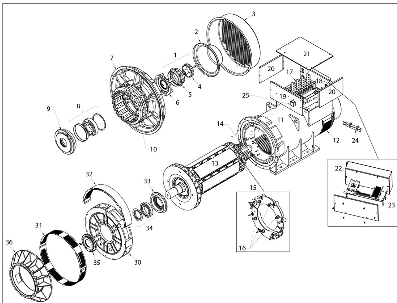
FIGURA 27. ALTERNATORE A7 A DUE CUSCINETTI
