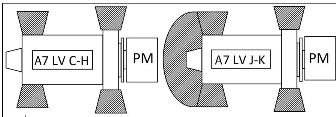
FIGURA 5. ZONE DI PERICOLO DELL'ALTERNATORE A BASSA TENSIONE A7
