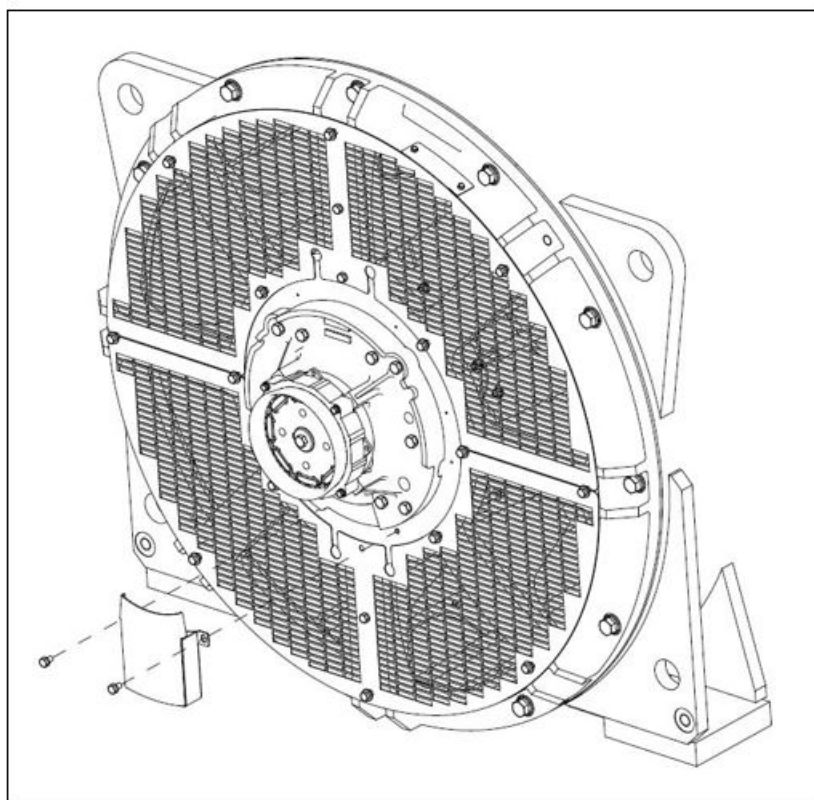
FIGURA 27. CONTENITORE DI RACCOLTA GRASSO S9
