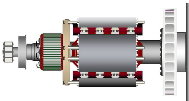
FIGURA 20. ROTORE DELL'ALTERNATORE A UN CUSCINETTO CHE MOSTRA I DISCHI DI ACCOPPIAMENTO IMBULLONATI AL MOZZO DI ACCOPPIAMENTO LATO CONDUTTORE (A DESTRA)
