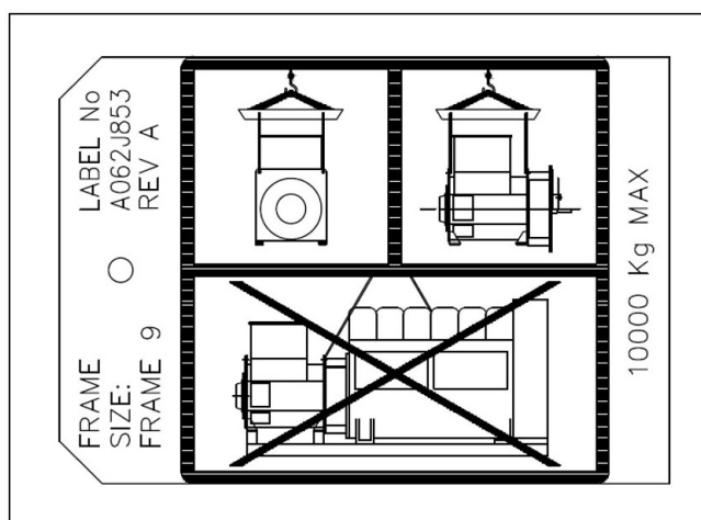
FIGURA 17. ESEMPIO DI ETICHETTA PER IL SOLLEVAMENTO
