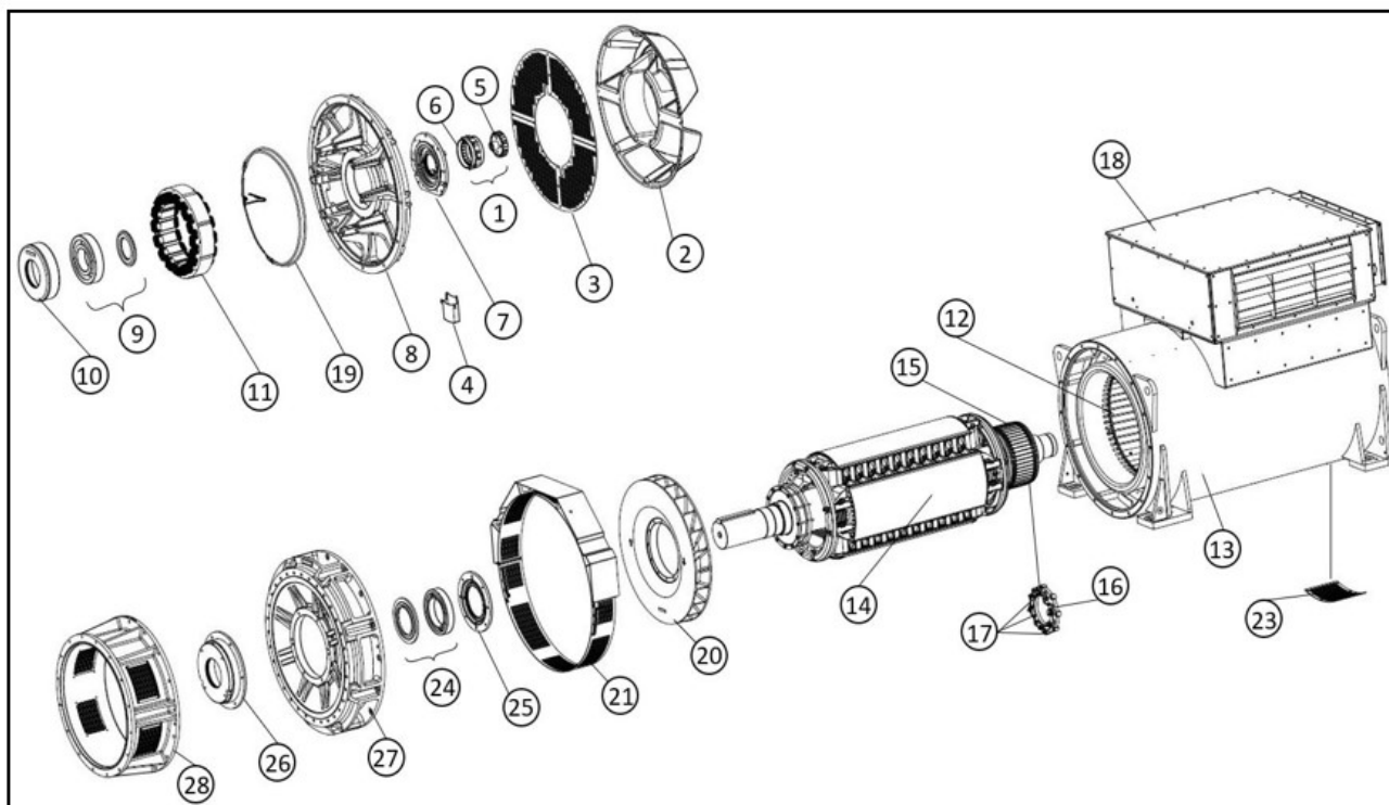
FIGURA 31. ALTERNADOR S9 DE BAJO VOLTAJE DE DOS COJINETES
