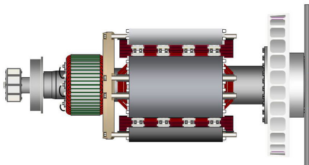
FIGURA 20. ROTOR DEL ALTERNADOR DE UN COJINETE EN EL QUE SE OBSERVAN LOS DISCOS DE ACOPLAMIENTO ATORNILLADOS AL CUBO DE ACOPLAMIENTO DEL EXTREMO IMPULSOR (A LA DERECHA)
