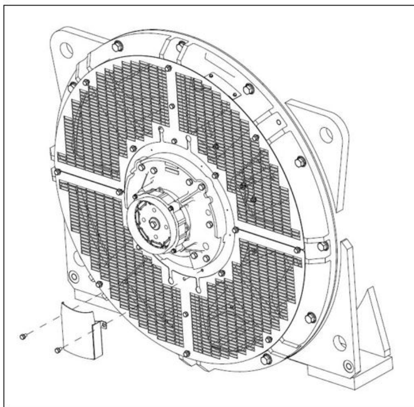
FIGURA 27. TRAMPA DE GRASA DE S9
