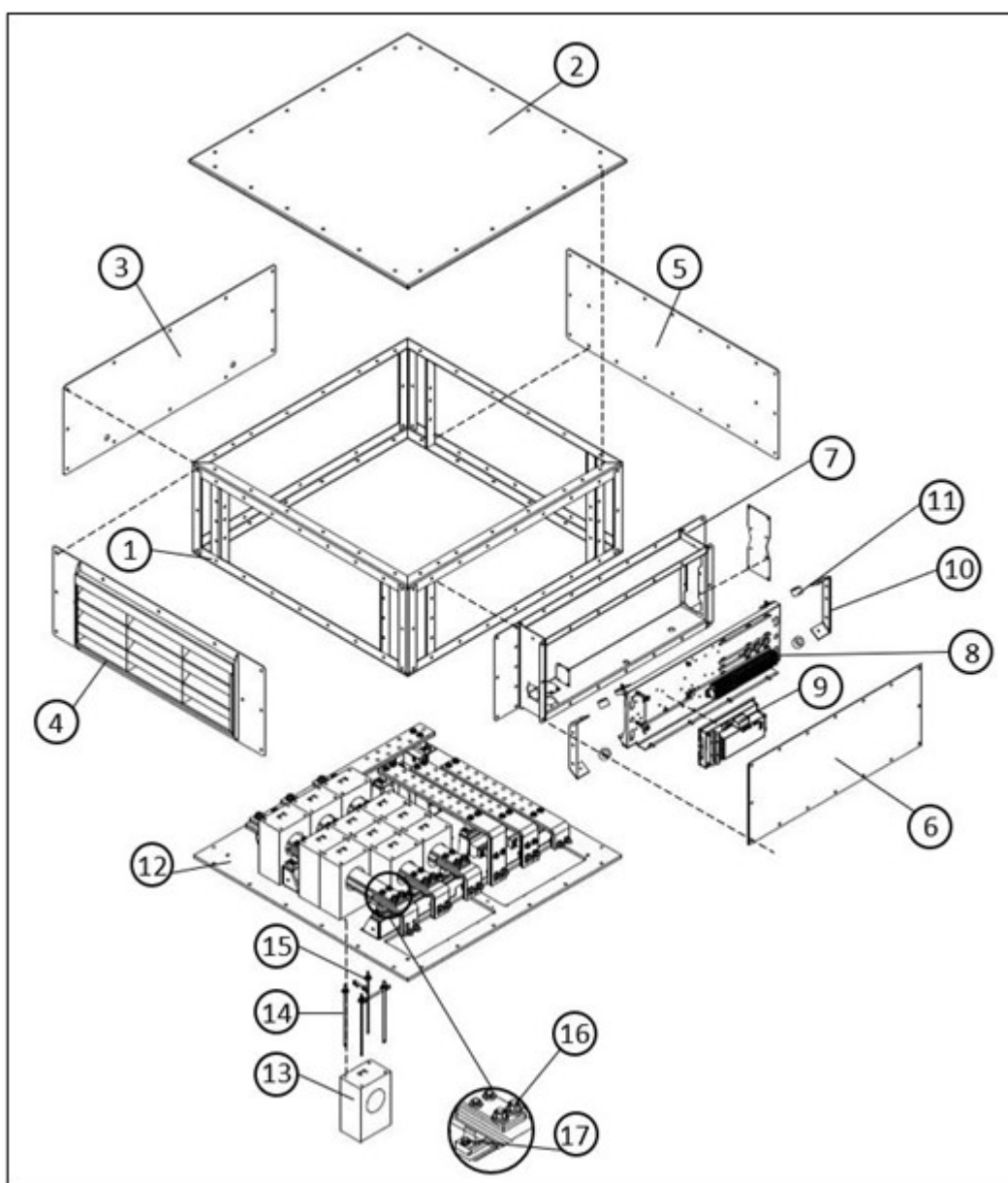
FIGURA 32. CAJA DE BORNES DE S9 DE BAJO VOLTAJE
