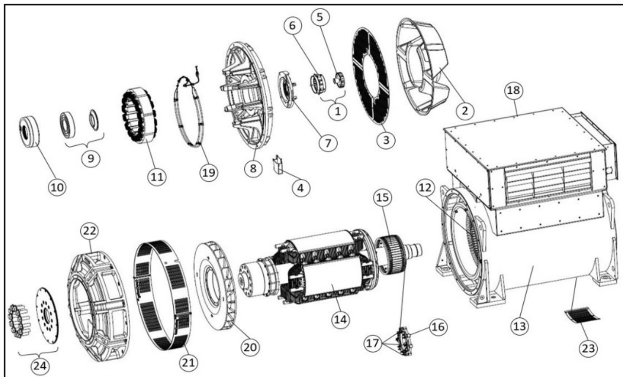
FIGURA 30. ALTERNADOR S9 DE BAJO VOLTAJE DE UN COJINETE
