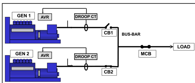
FIGUR 26. PARALLELLA ELLER SYNKRONISERANDE VÄXELSTRÖMSGENERATORER
