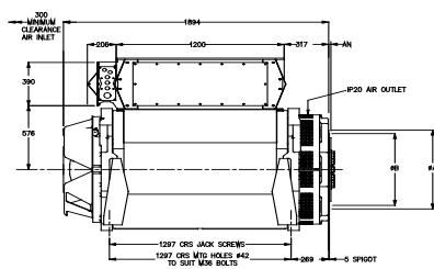
P80 R/S/T CORES
