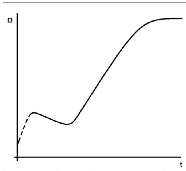
図 19. 絶縁抵抗のグラフ
