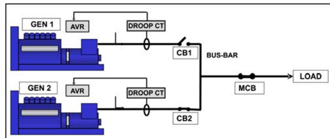
図 17. オルタネーターの並列運転または同期化
