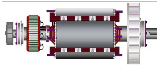
図 14. 2 ベアリング オルタネーターの回転子: 右側にフレキシブル結合用のキー溝の付いたシャフトがある
