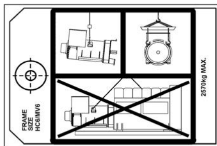
図 11. 吊り上げラベル
