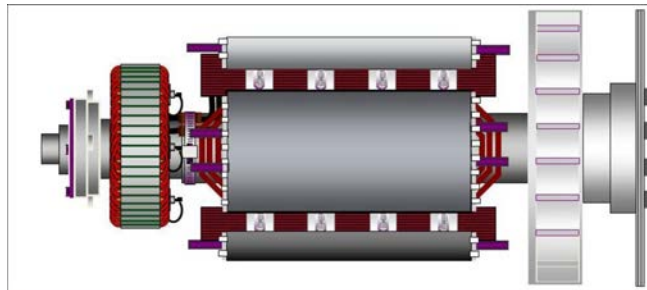
図 13. 1 ベアリング オルタネーターの回転子: カップリング ディスクが右側の駆動側カップリング ハブにボルトで固定されている
