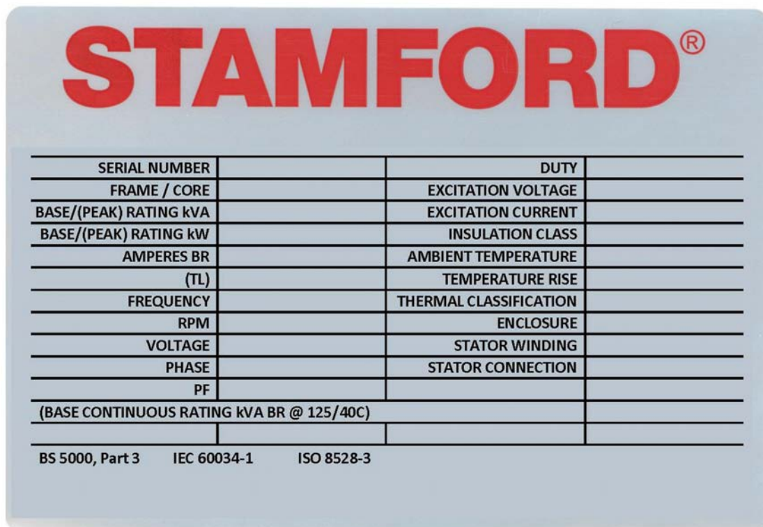
FIGURE 1. PLAQUE SIGNALÉTIQUE DES ALTERNATEURS C.A. GLOBAL STAMFORD
