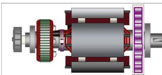
FIGURE 6. ROTOR DE L'ALTERNATEUR À PALIER DOUBLE MONTRANT L'ARBRE AVEC CLAVETTE POUR ACCOUPLEMENT FLEXIBLE (À DROITE)
