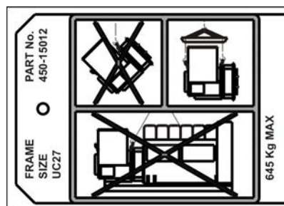
FIGUR 4. LYFTDEKAL
