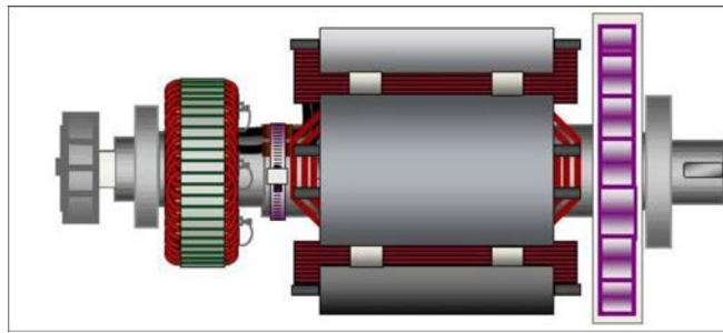
FIGUR 6. ROTORN I EN VÄXELSTRÖMSGENERATOR MED TVÅ LAGER SOM VISAR AXEL MED KILSPÅR FÖR FLEXIBEL KOPPLING (TILL HÖGER)
