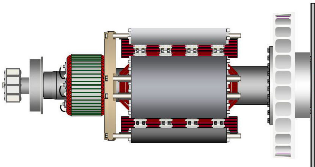
图 9. 显示锚固到驱动端耦合集线器的耦合盘（右侧）的单轴承交流发电机
