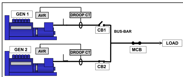
图 14. 并联或同步交流发电机
