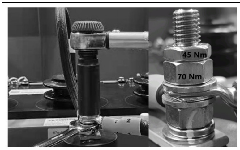
图 13. 夹紧正确的线缆（多条线缆）
