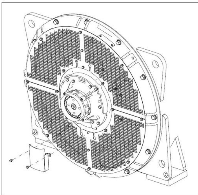
图 15. 润滑脂捕集器 P80D
