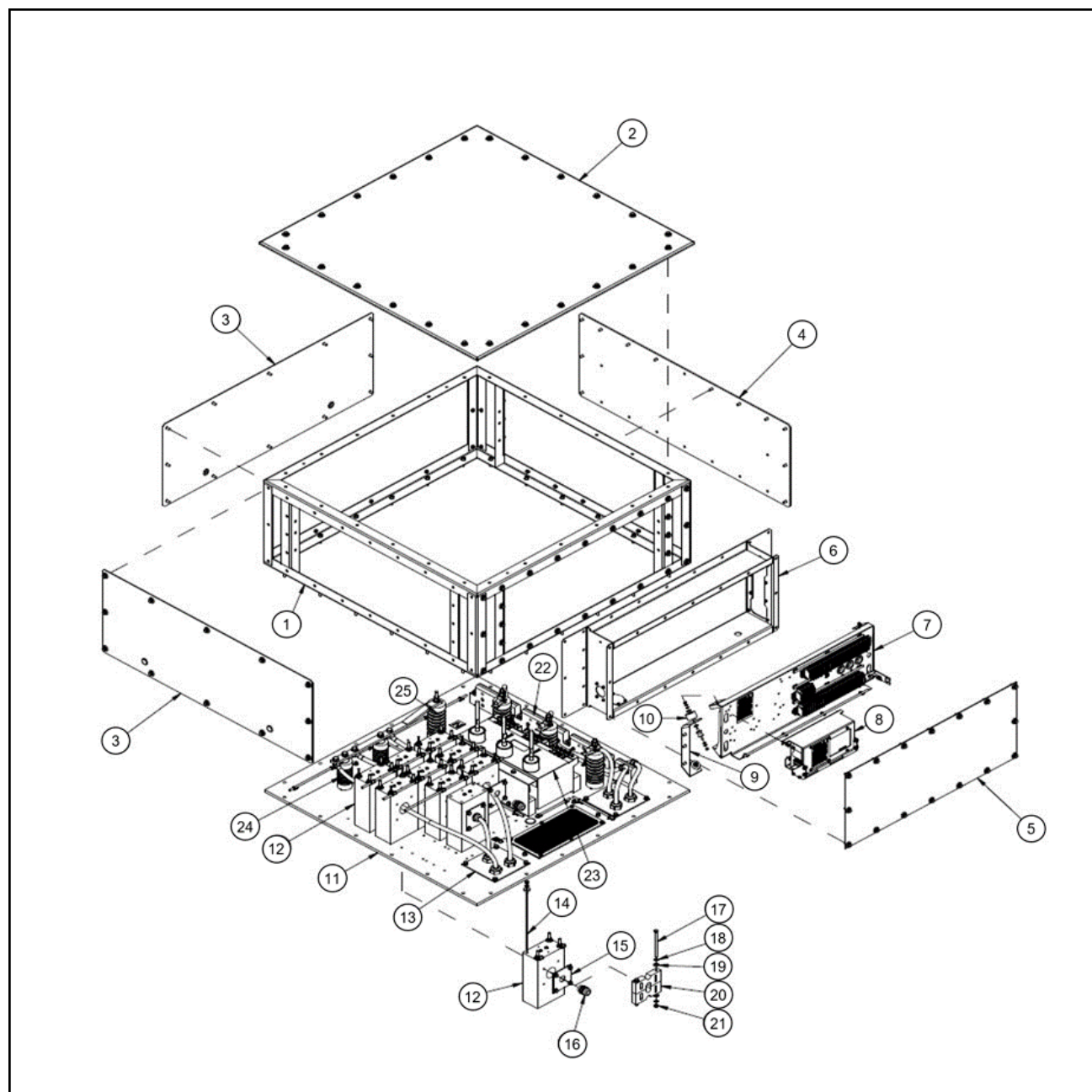
图 19. P80D HV 接线盒
