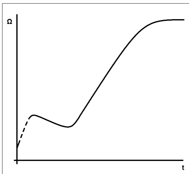
图 17. 绝缘电阻图
