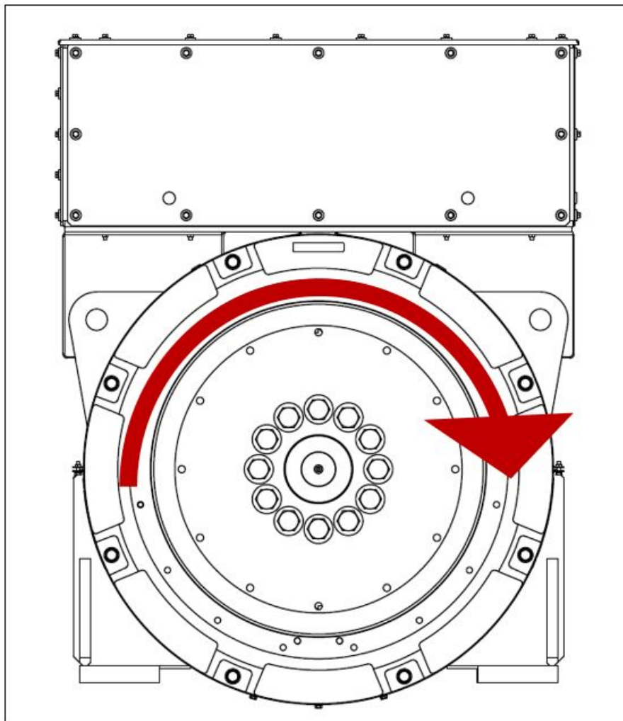
图 12. 旋转方向
