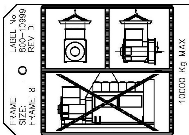
图 7. 起吊标签
