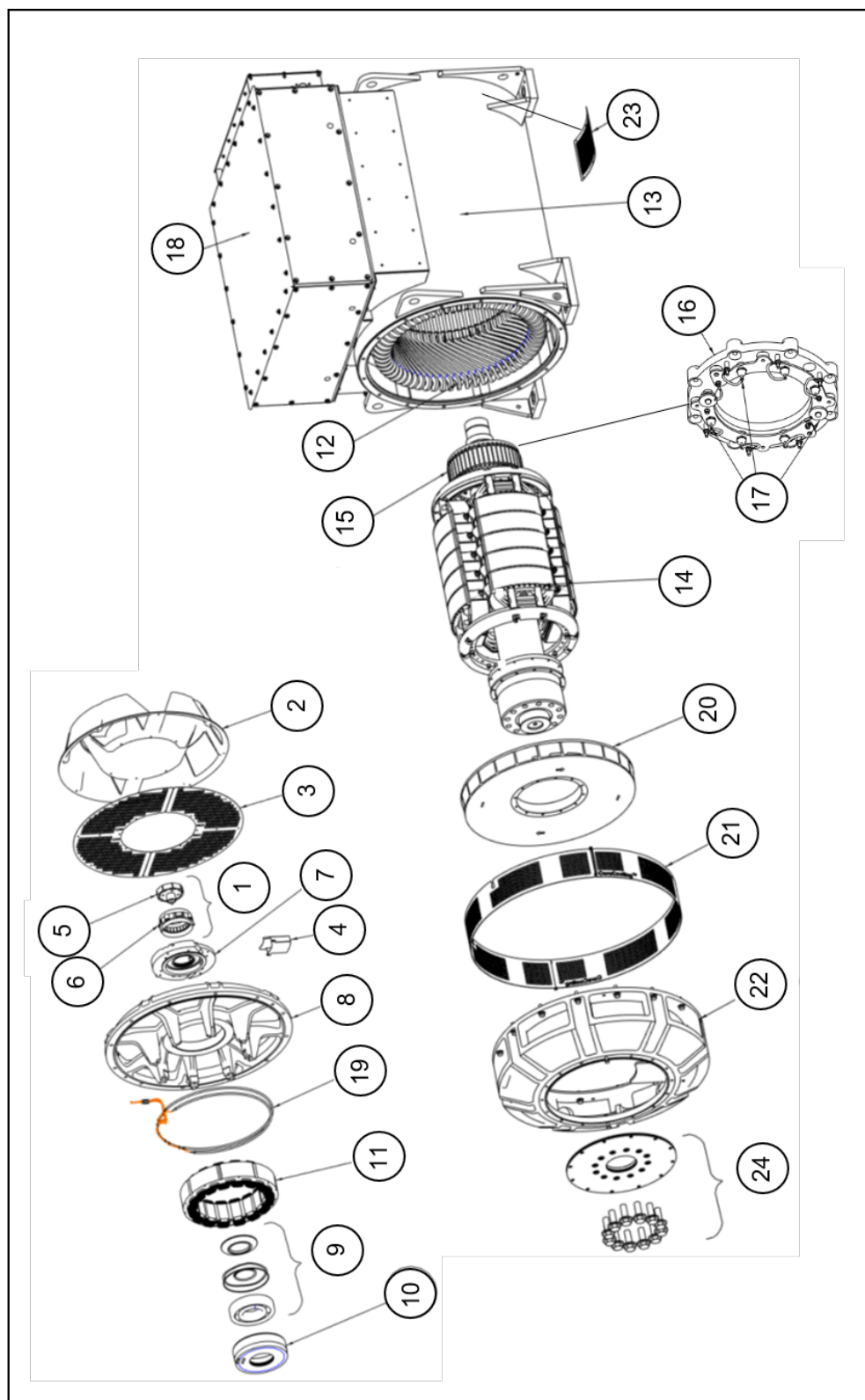
图 18. P90D 单轴承交流发电机
