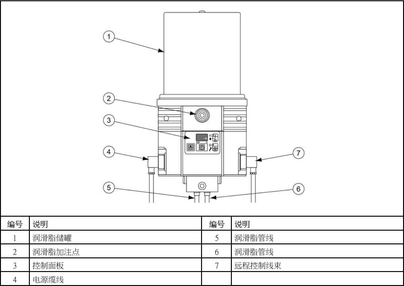
图 9. 典型自动交流发电机轴承再润滑器
