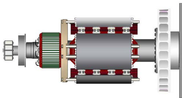
图 5. 显示锚固到驱动端耦合集线器的耦合盘（右侧）的单轴承交流发电机
