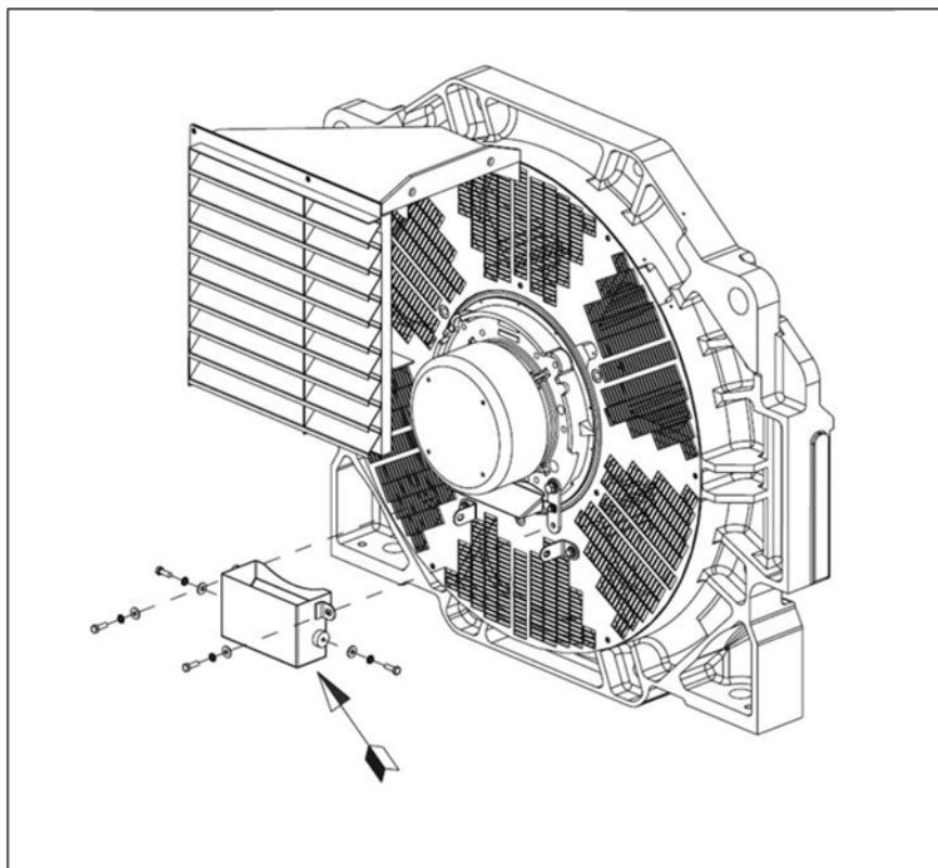
图 8. 带空气滤清器的 P80 交流发电机上的润滑脂捕集器
